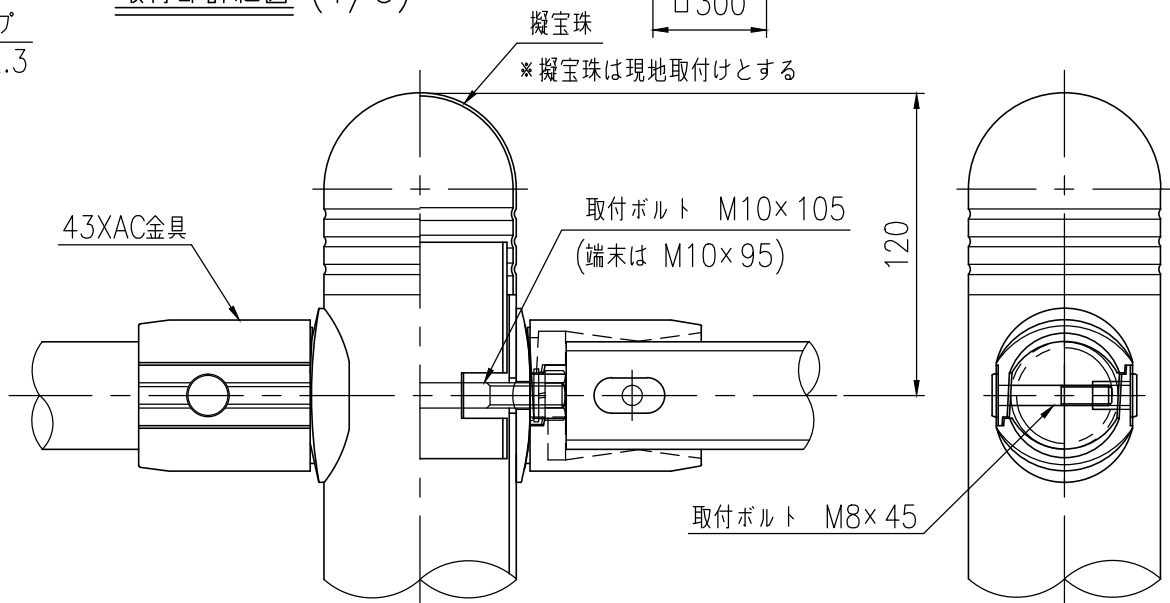
取付部詳細図 (1/3)
