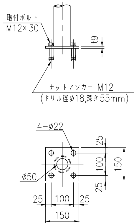
ベースプレート詳細図 (1/10)
