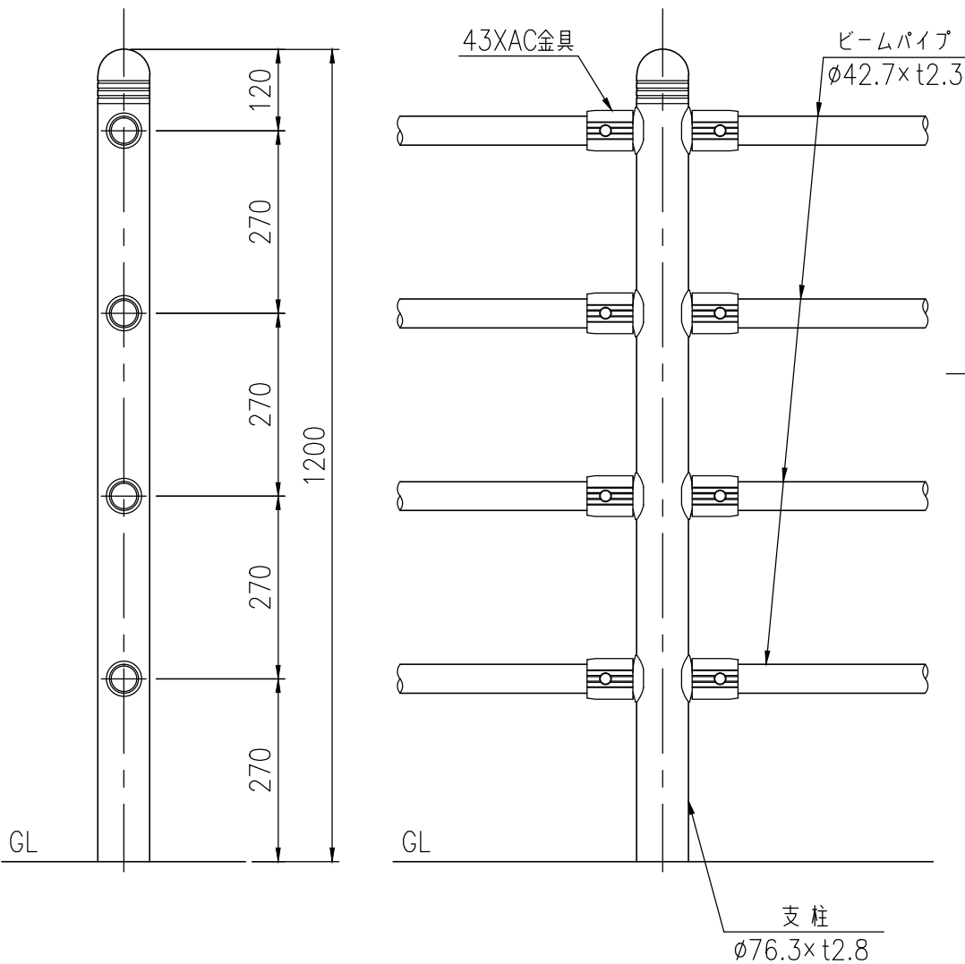
支柱図 (1/10)
