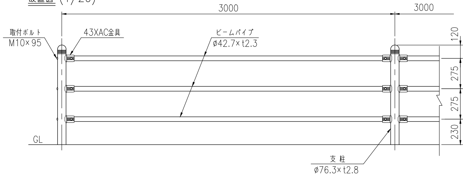
設置図 (1/20)
