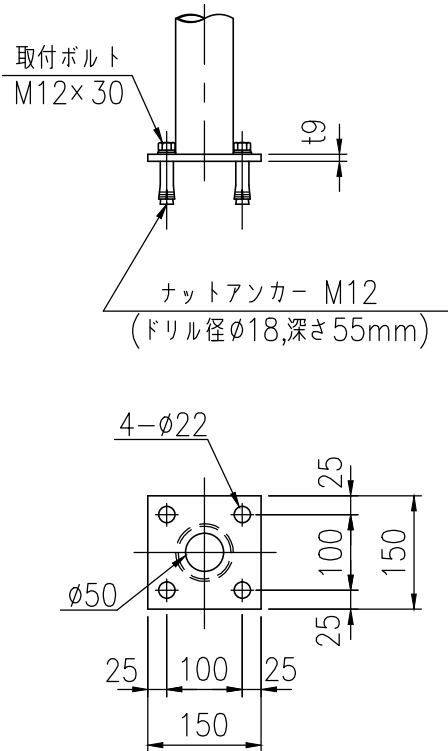
ベースプレート詳細図 (1/10)
