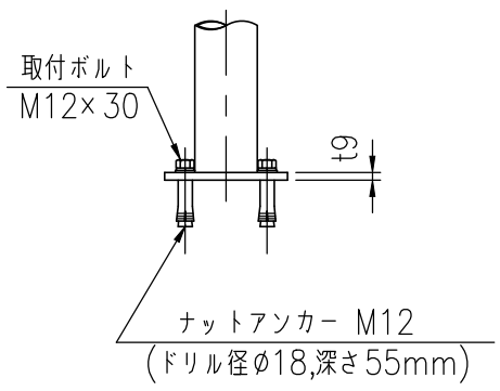
ベースプレート詳細図 (1/10)
