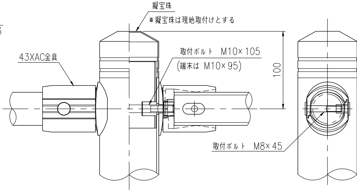
取付部詳細図 (1/3)
