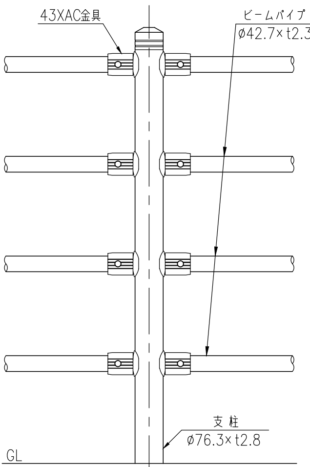
支柱図 (1/10)
