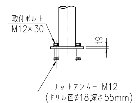
ベースプレート詳細図 (1/10)
