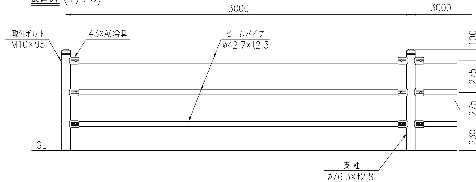
設置図 (1/20)
