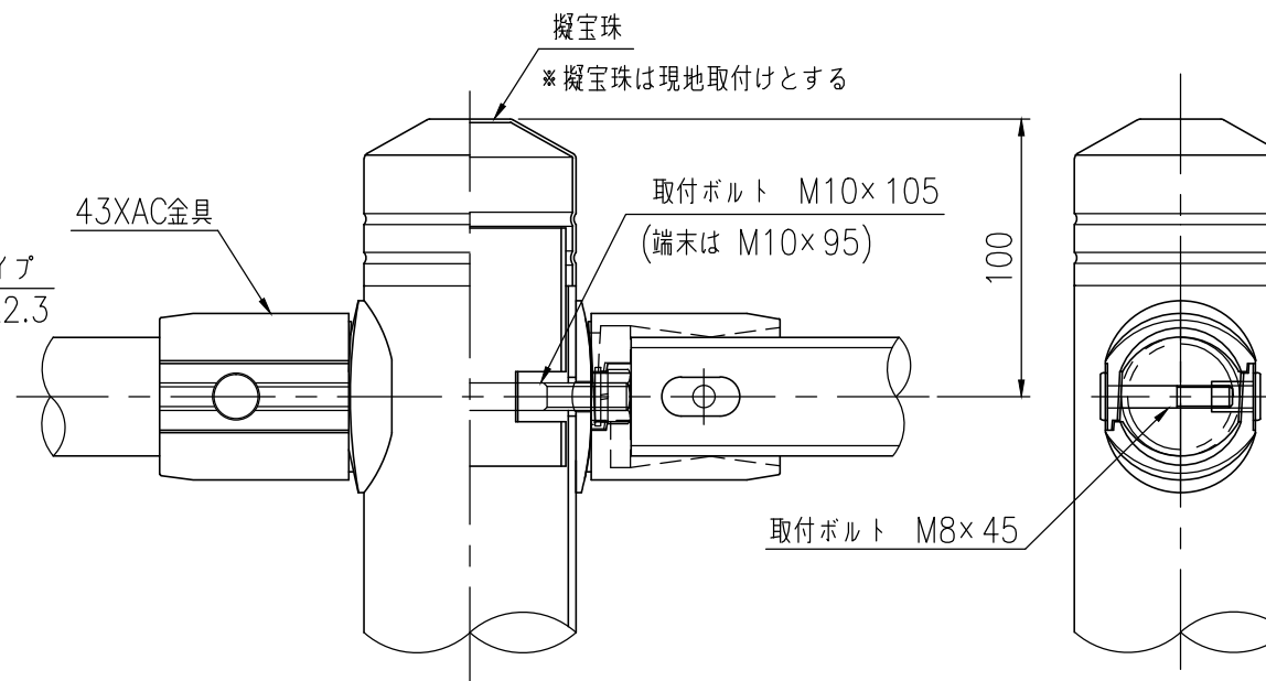
取付部詳細図 (1/3)
