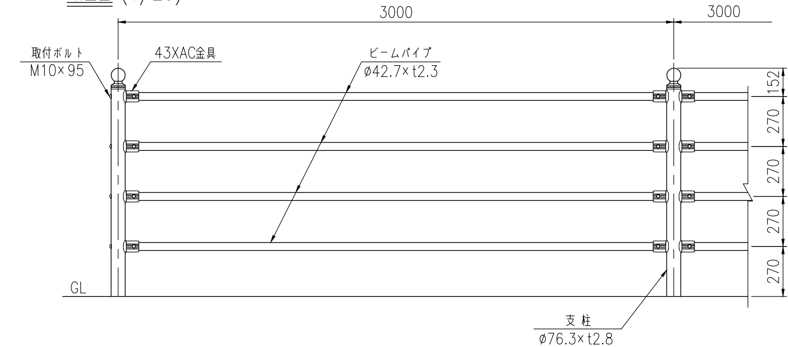
支柱図 (1/10)
