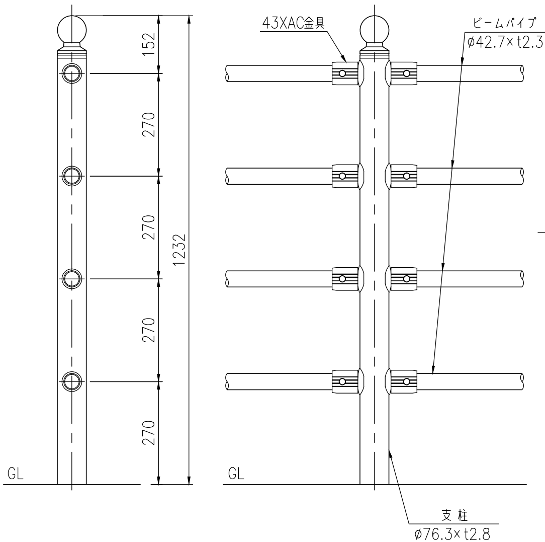
支柱図 (1/10)
