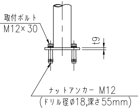
ベースプレート詳細図 (1/10)
