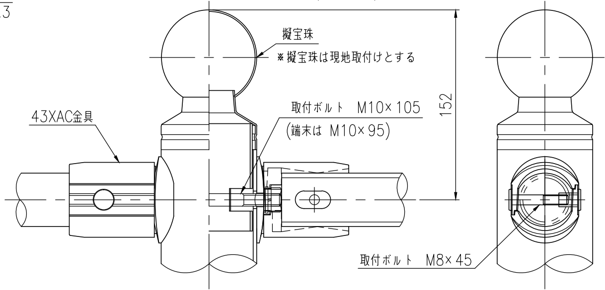
取付部詳細図 (1/3)
