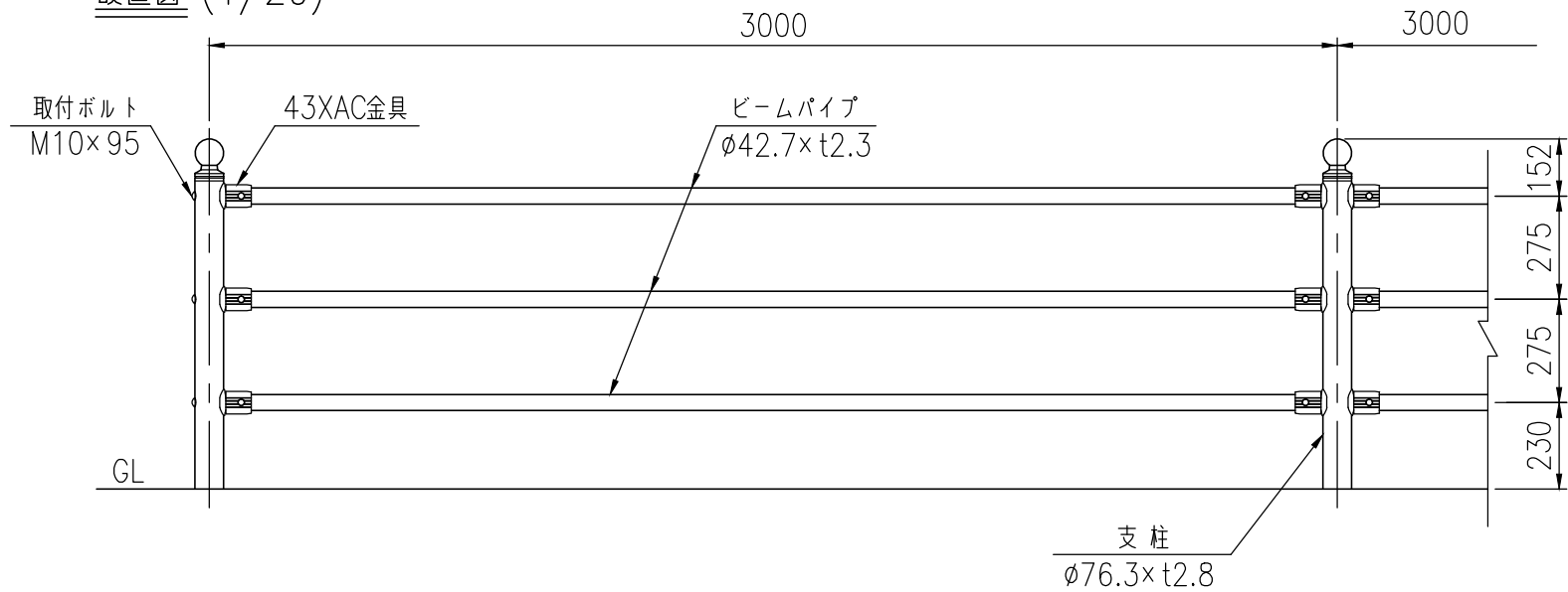
設置図 (1/20)
