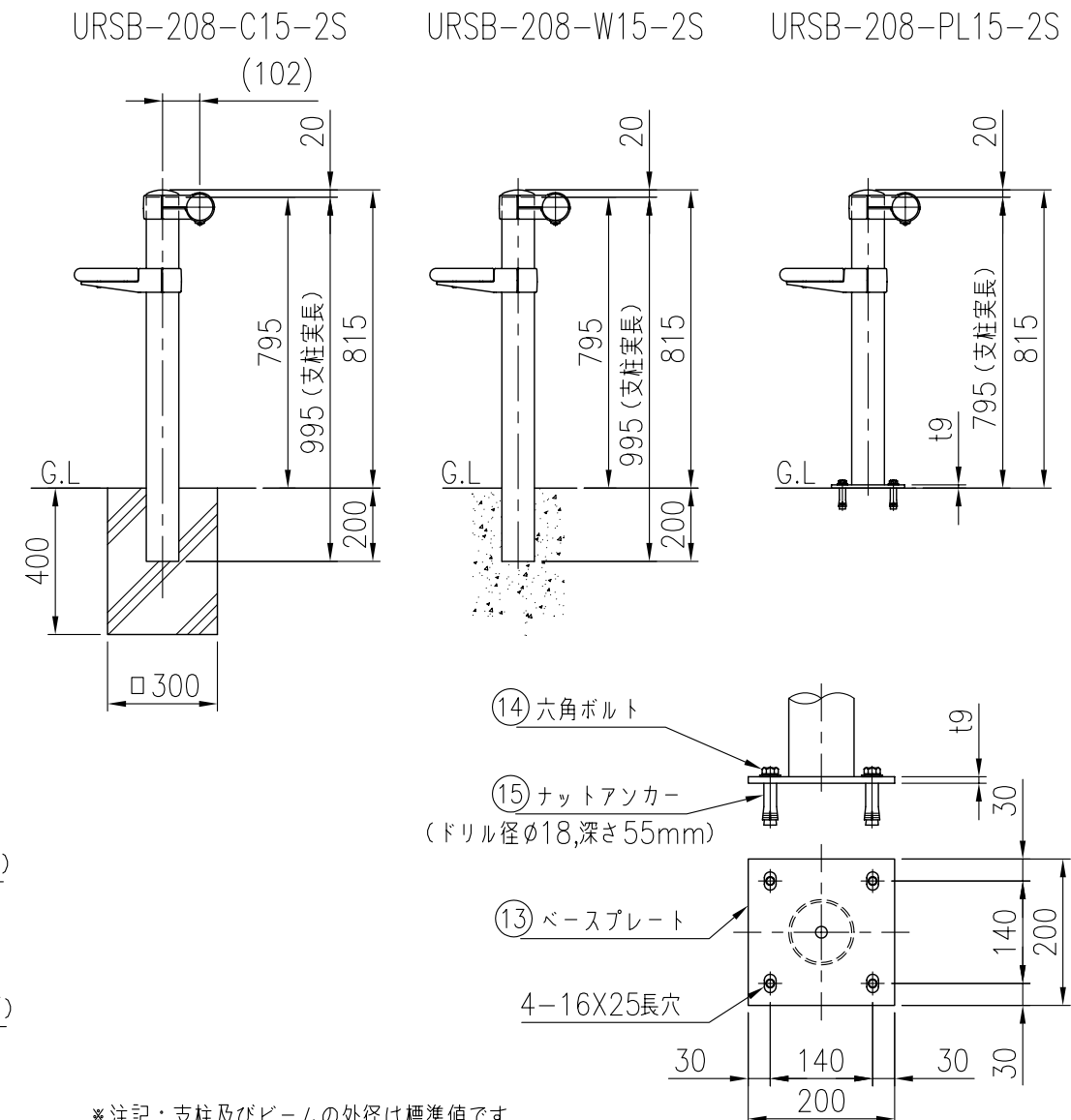
ベースプレート詳細図 (1 / 10)
