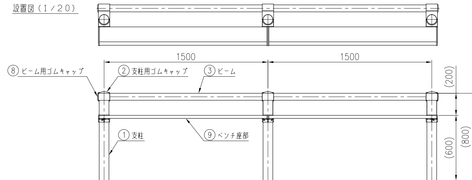
取付部詳細図 (1 / 5)
