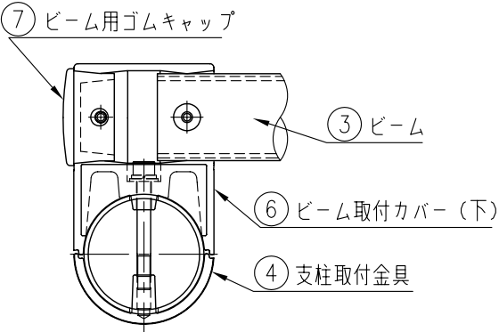
取付部詳細図 ( 1 / 5 )
