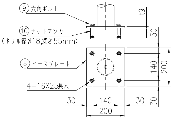
ベースプレート詳細図（1 / 10）
