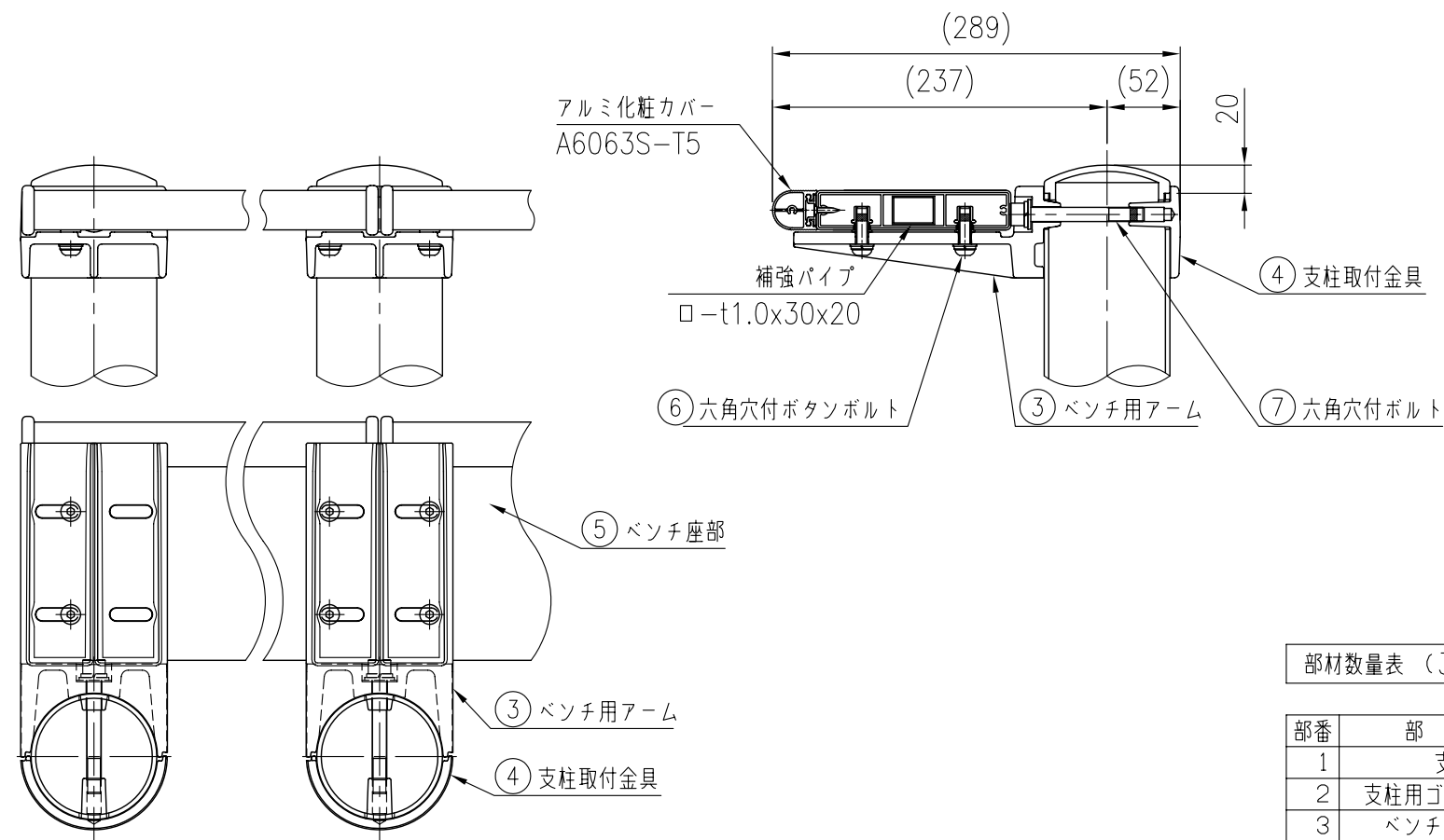
取付部詳細図（1 / 5）
