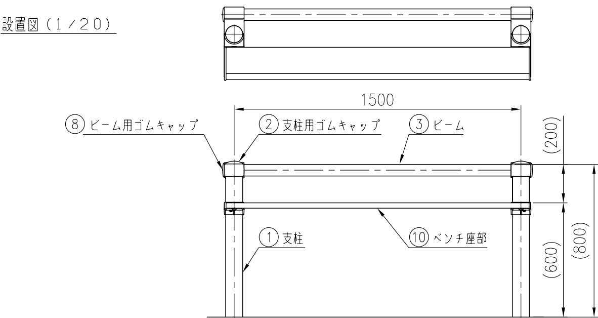
取付部詳細図 (1 / 5)
