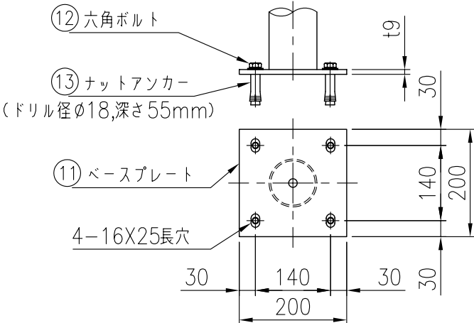
ベースプレート詳細図（1 / 1 0）
