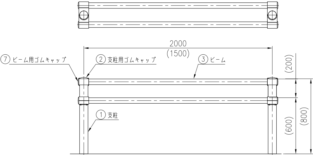
設置図（1 / 2 0）
