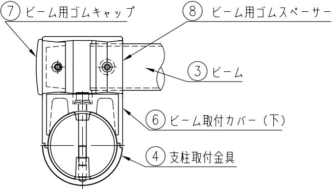
取付部詳細図（1 / 5）
