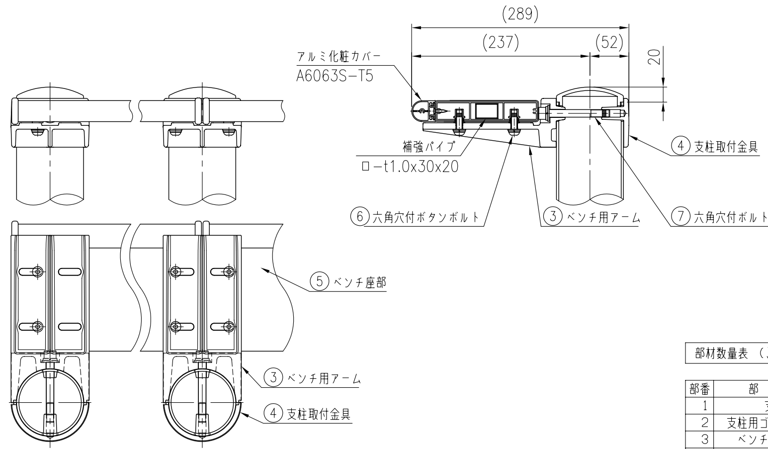
取付部詳細図 ( 1 / 5 )
