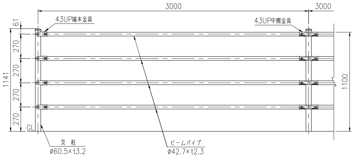
設置図 (1/20)
