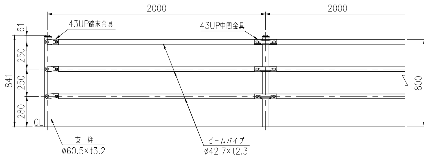
設置図 (1/20)
