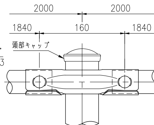
取付部詳細図 (1/4)
