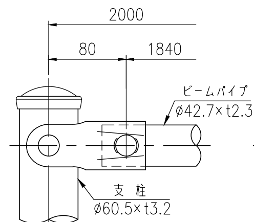
取付部詳細図 (1/4)
