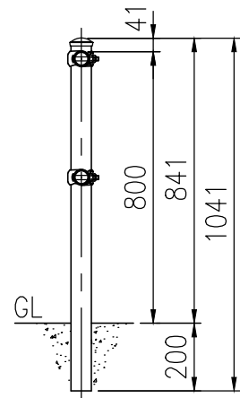
UP-208W30
