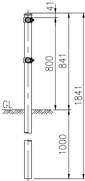
UP-208E30
