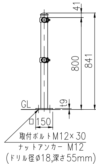
UP-208PL30
