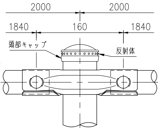
取付部詳細図 (1/4)
