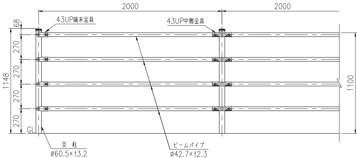
設置図 (1/20)
