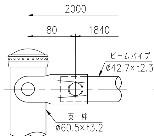
取付部詳細図 (1/4)
