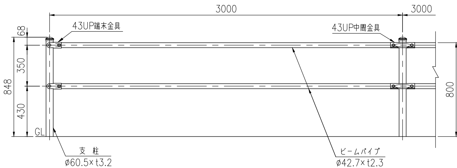
設置図 (1/20)
