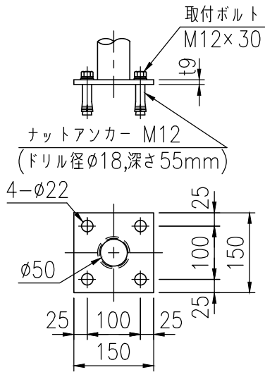
ベースプレート詳細図 (1/10)
