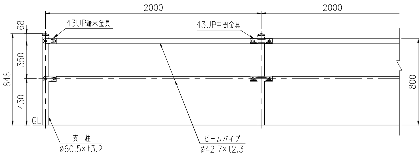
設置図 (1/20)
