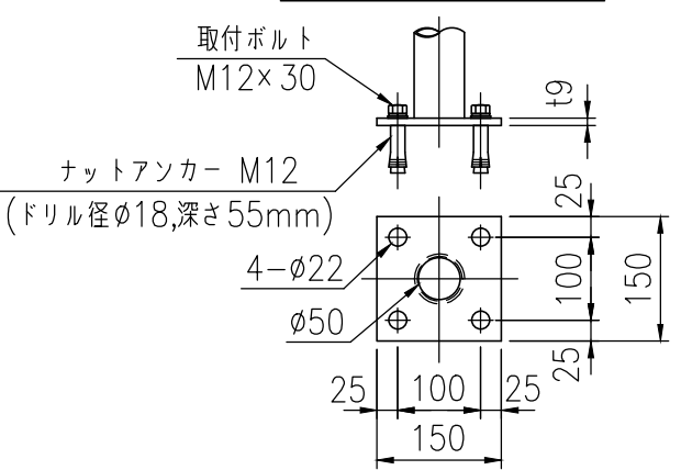
ベースプレート詳細図 (1/10)
