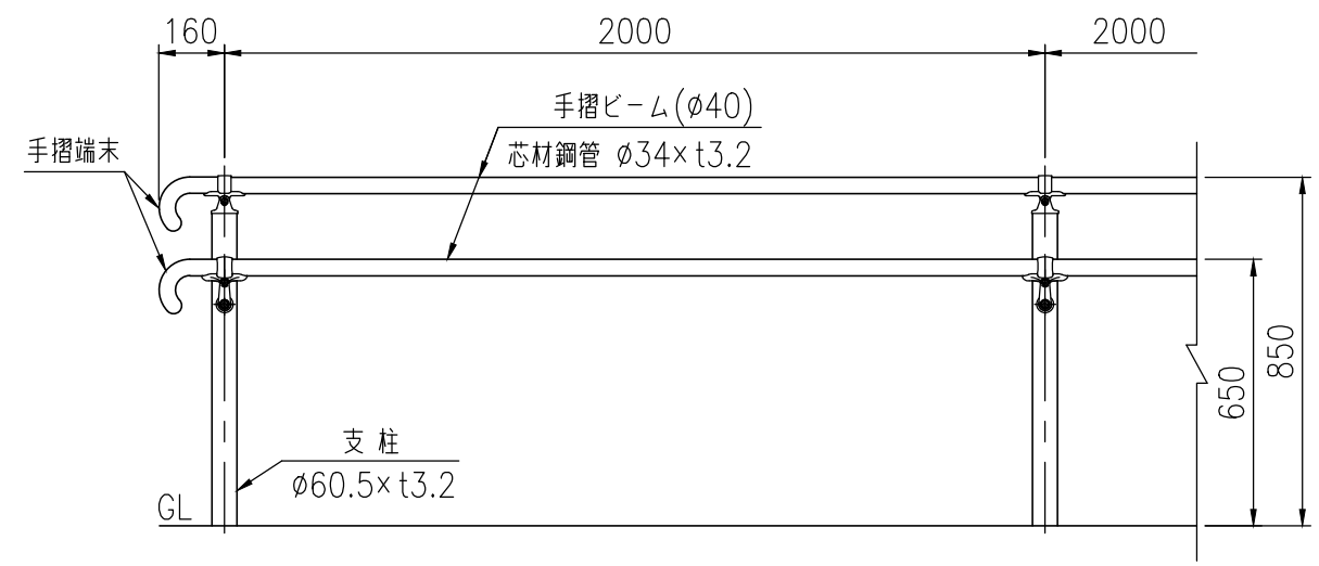
支柱図 (1/10)
