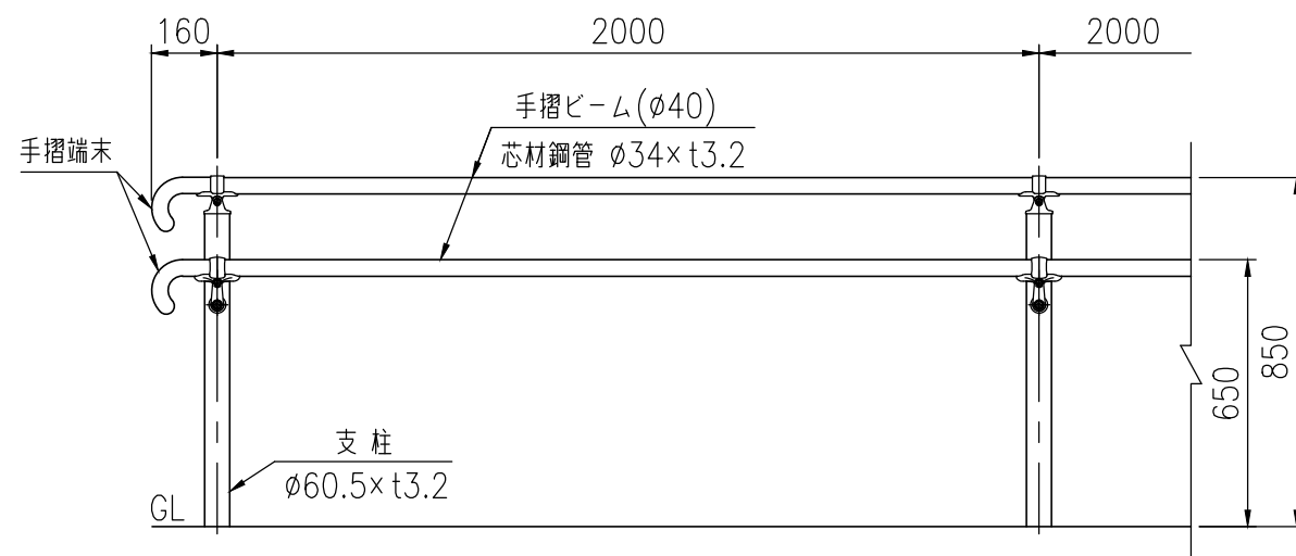
支柱図 (1/10)
