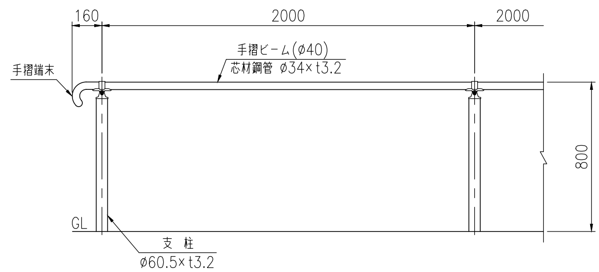
設置図 (1/20)
