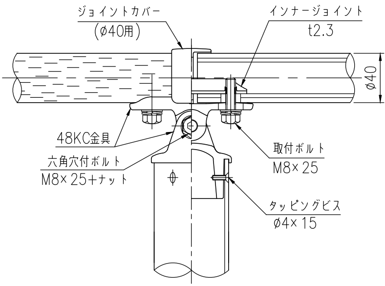
取付部詳細図 (1/3)
