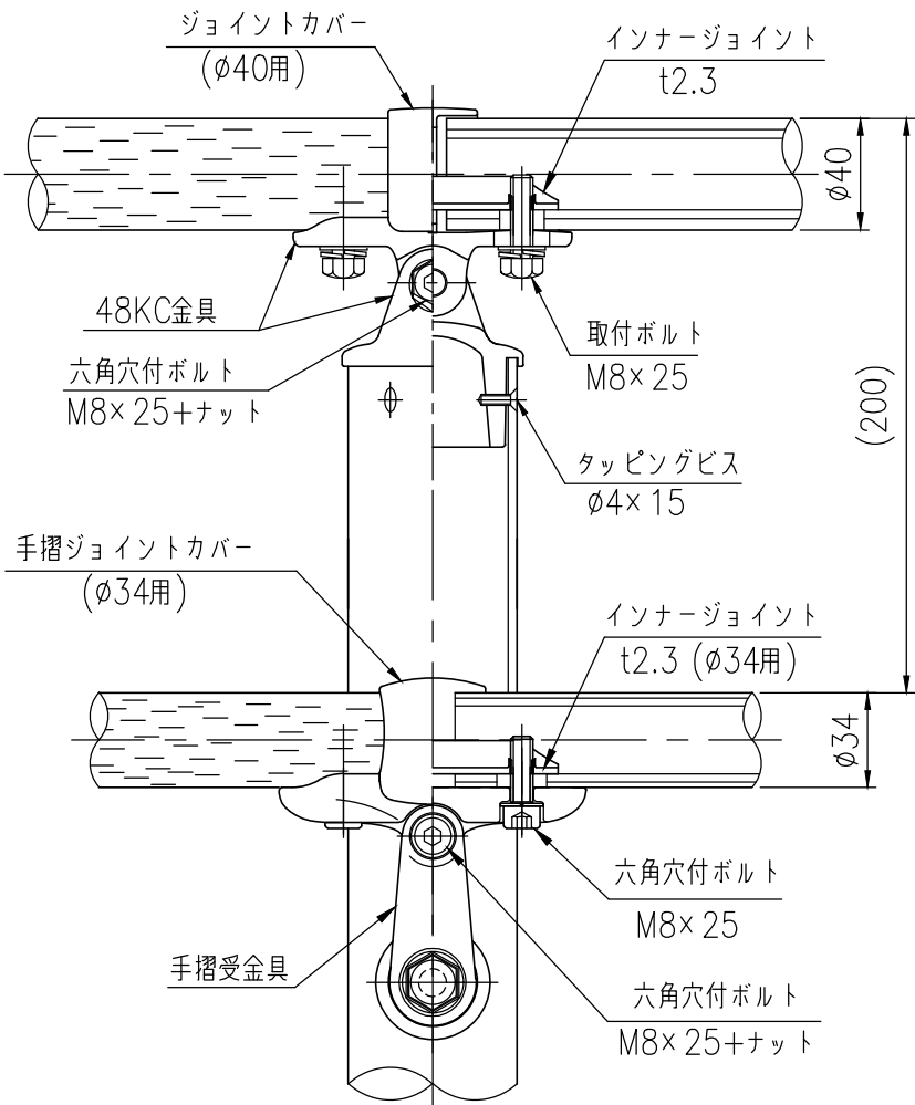
取付部詳細図 (1/3)
