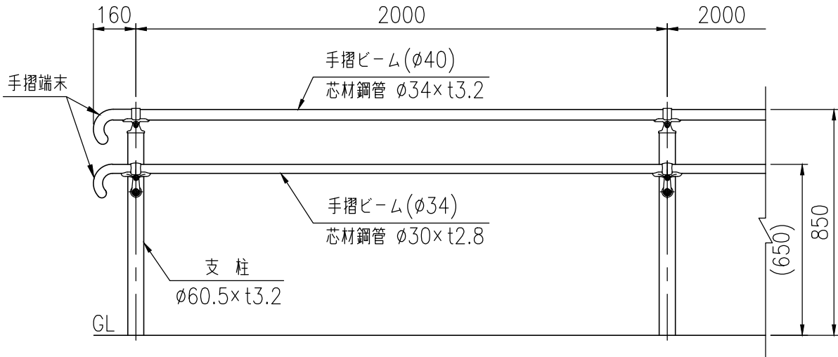
支柱図 (1/10)
