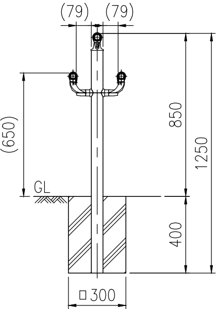
取付部詳細図 (1/3)
