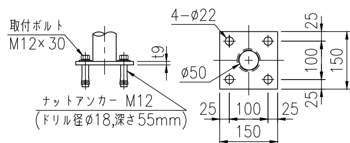
ベースプレート詳細図 (1/10)
