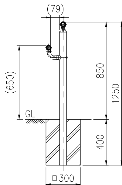
取付部詳細図 (1/3)
