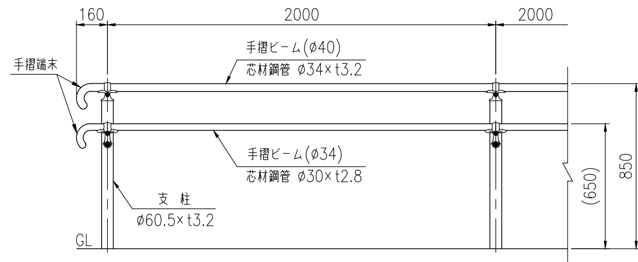
支柱図 (1/10)
