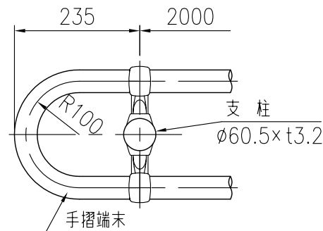
手摺端末平面図 (1/10)
