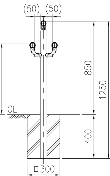
支柱図 (1/10)
