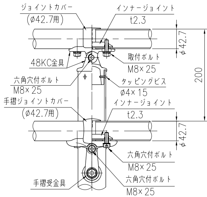
取付部詳細図 (1/5)
