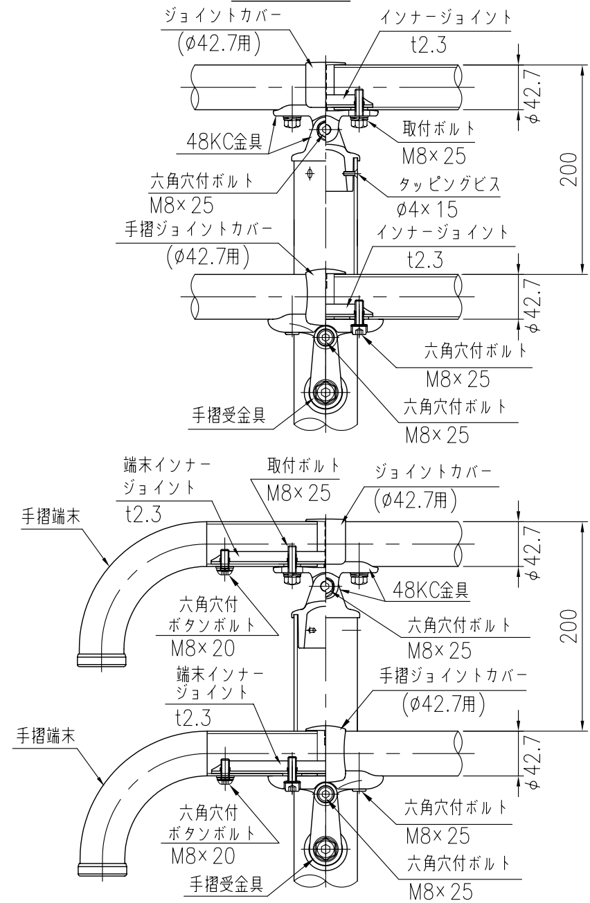
取付部詳細図 (1/5)
