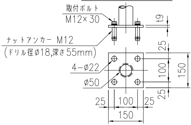
ベースプレート詳細図 (1/10)
