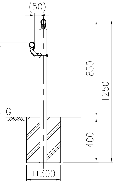
支柱図 (1/10)
