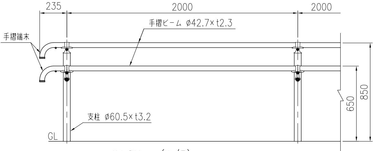
取付部詳細図 (1/5)
