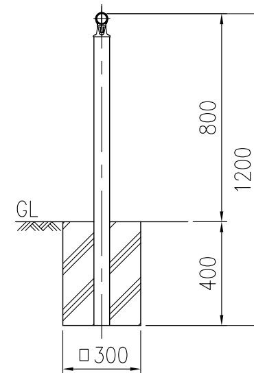
支柱図 (1/10)
