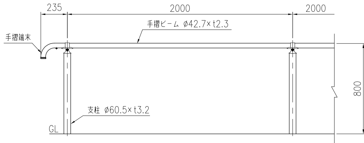
設置図 (1/20)
