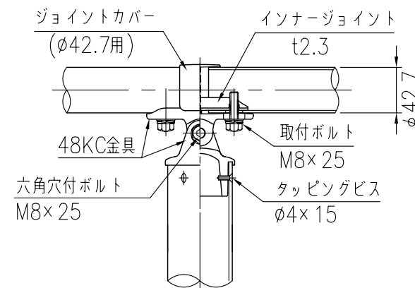
取付部詳細図 (1/5)
