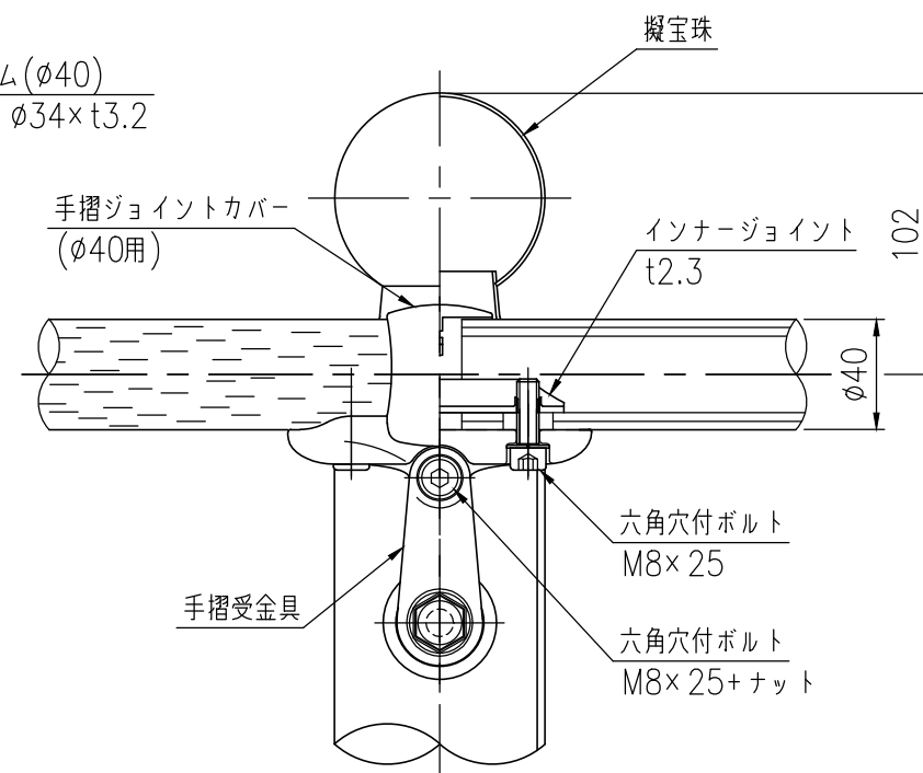
取付部詳細図 (1/3)
