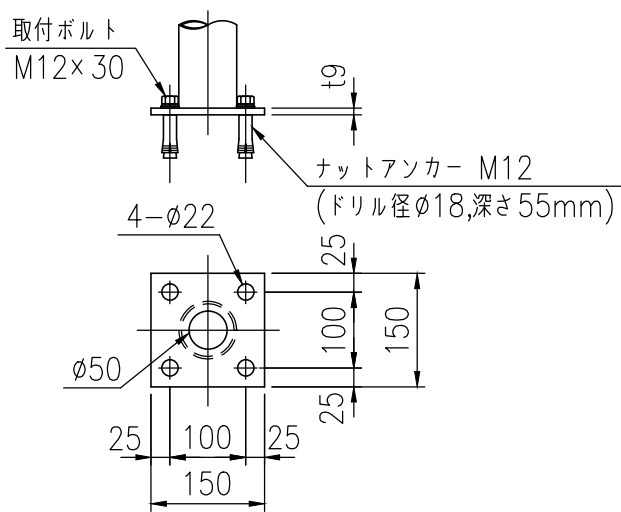
ベースプレート詳細図 (1/10)
