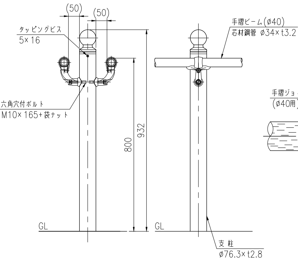
支柱図 (1/10)
