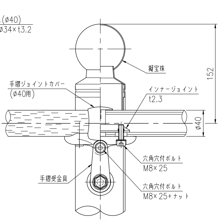
取付部詳細図 (1/3)
