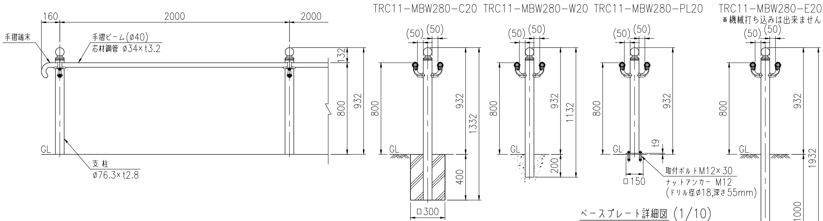
支柱図 (1/10)
