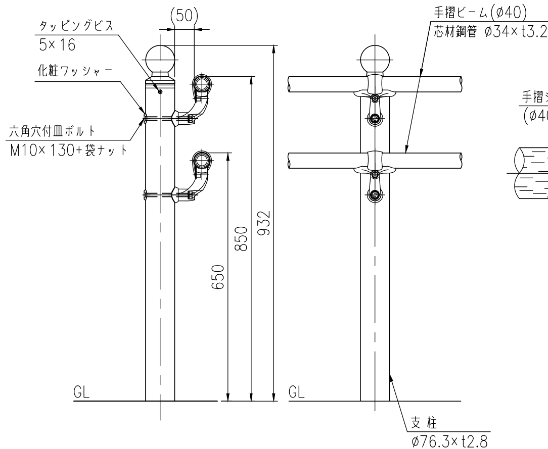
支柱図 (1/10)
