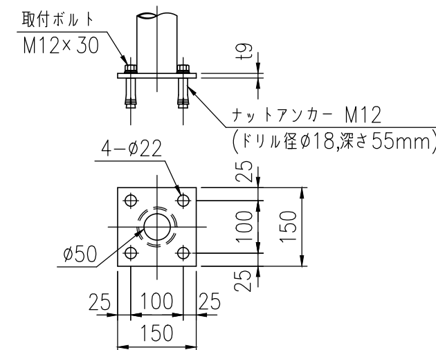
ベースプレート詳細図 (1/10)
