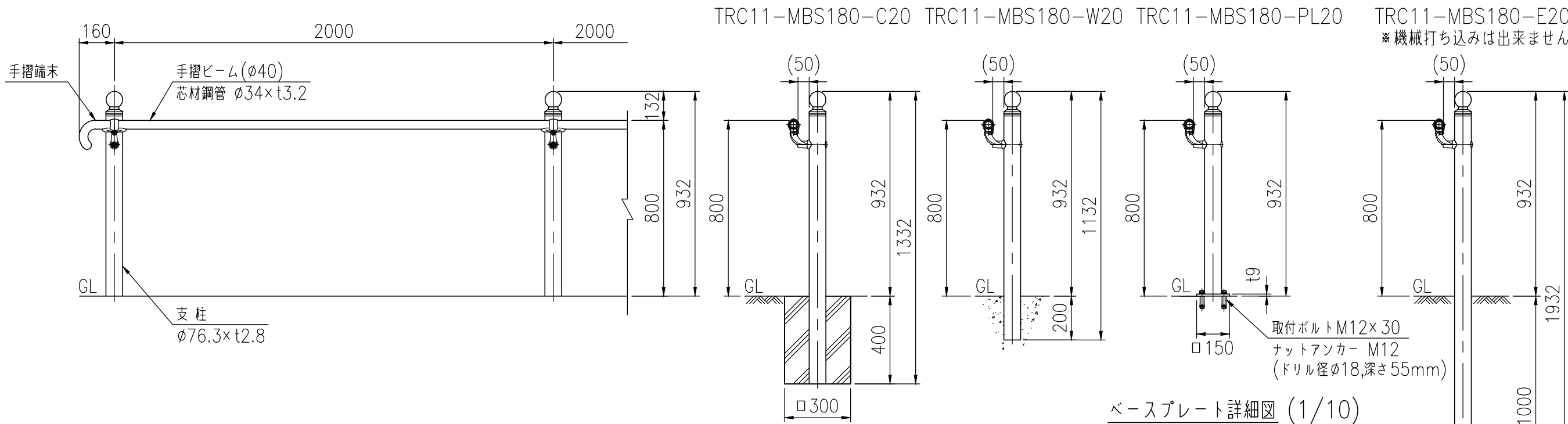
支柱図 (1/10)
