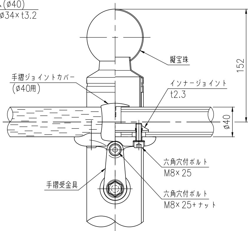
取付部詳細図 (1/3)
