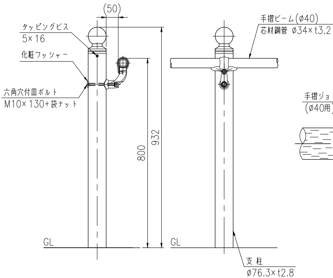
支柱図 (1/10)
