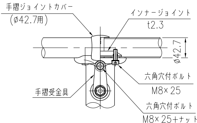
取付部詳細図 (1/5)
