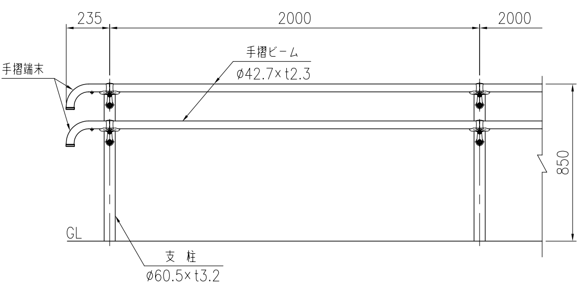
設置図 (1/20)
