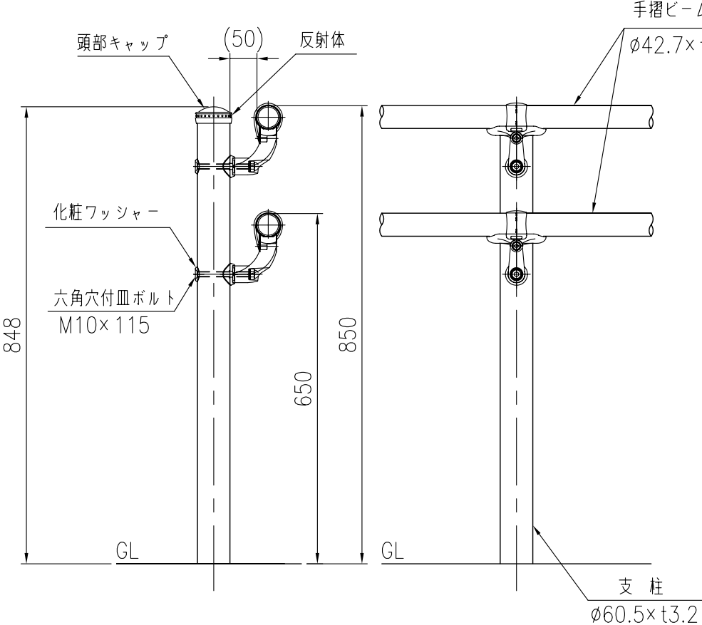
支柱図 (1/10)
