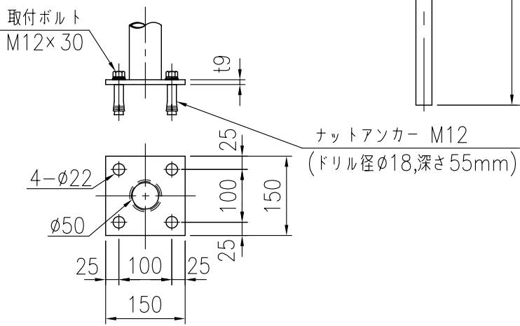
ベースプレート詳細図 (1/10)
