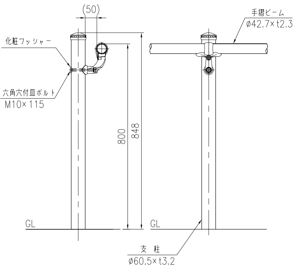
支柱図 (1/10)
