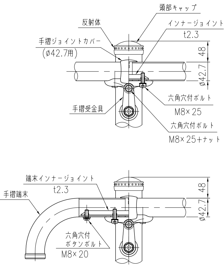
取付部詳細図 (1/5)
