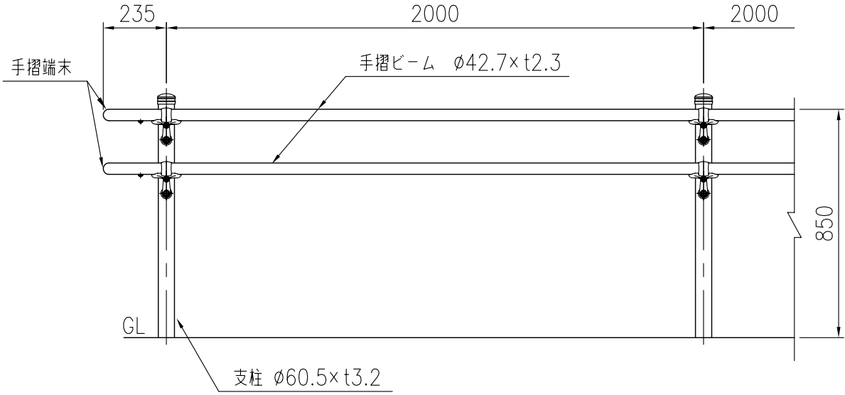
設置図 (1/20)
