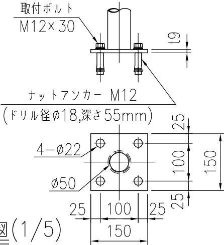
ベースプレート詳細図 (1/10)
