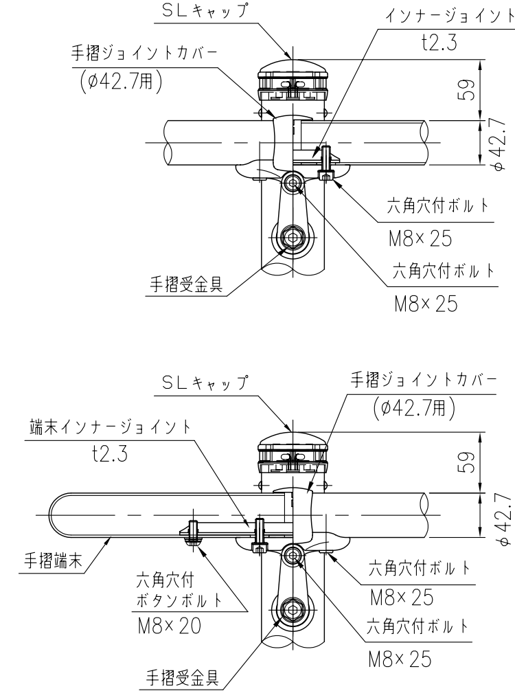
取付部詳細図 (1/5)
