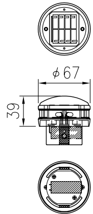
SLキャップ詳細図 (1/5)
