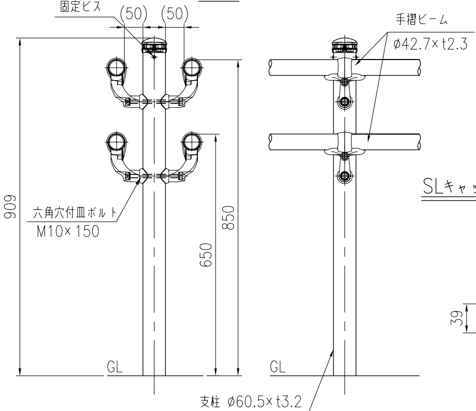
支柱図 (1/10)
