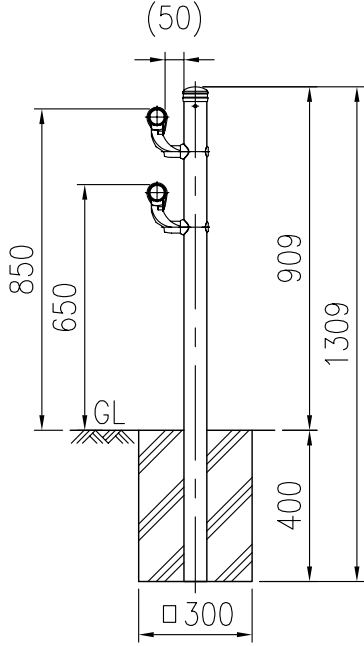
支柱図 (1/10)
