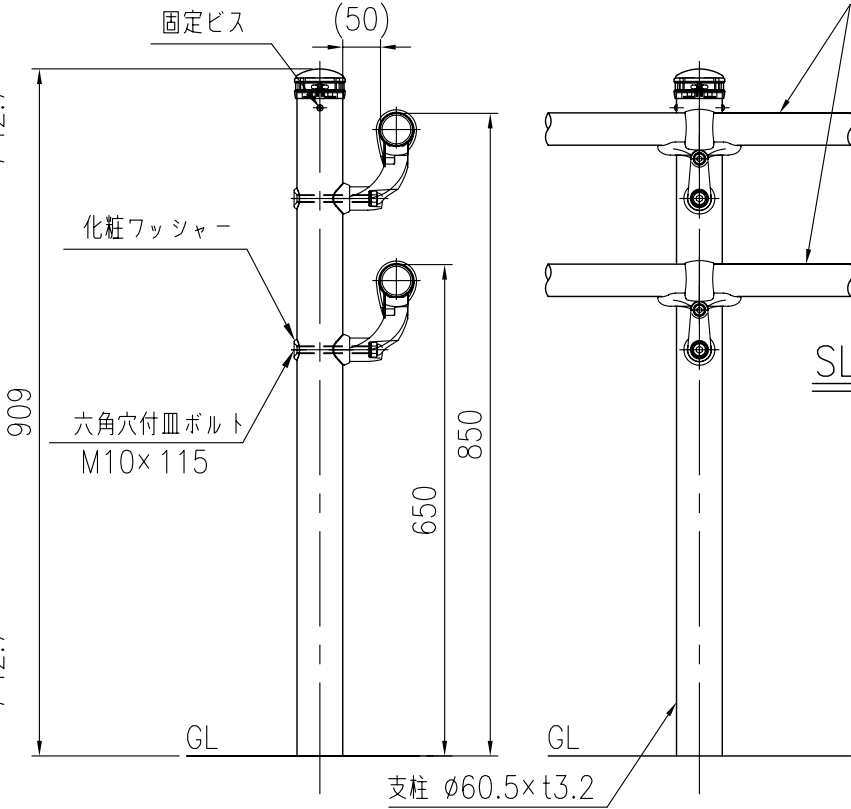
支柱図 (1/10)
