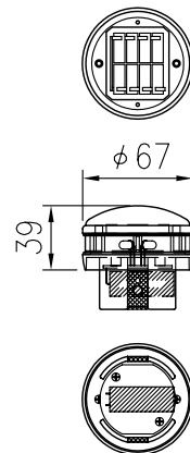
SLキャップ詳細図 (1/5)
