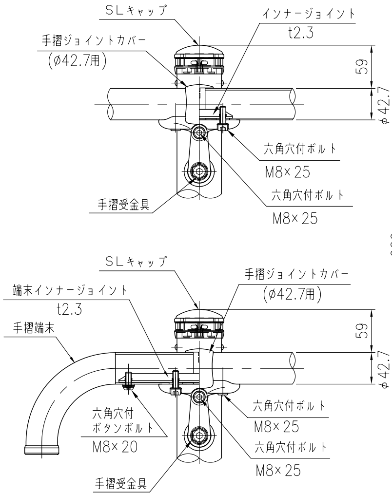
取付部詳細図 (1/5)
