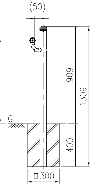
支柱図 (1/10)
