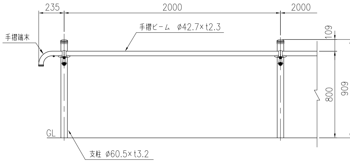
設置図 (1/20)
