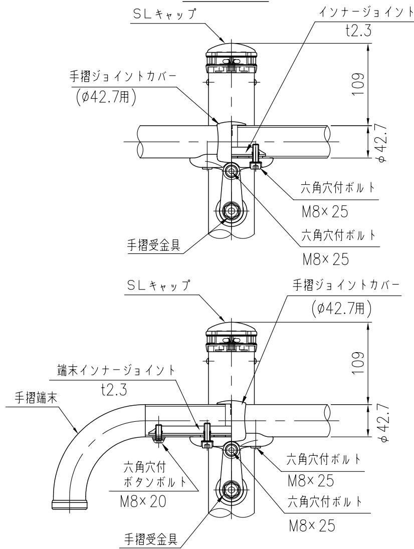
取付部詳細図 (1/5)
