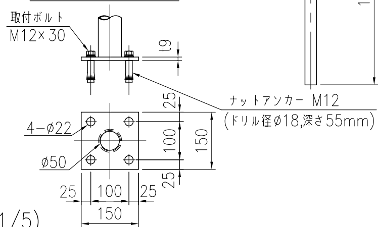
ベースプレート詳細図 (1/10)
