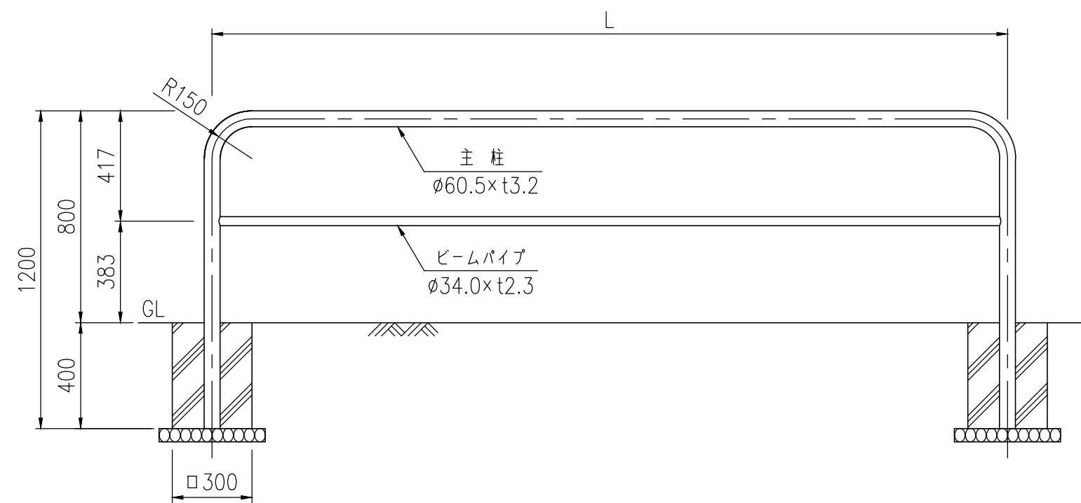
設置図 (1/20)
