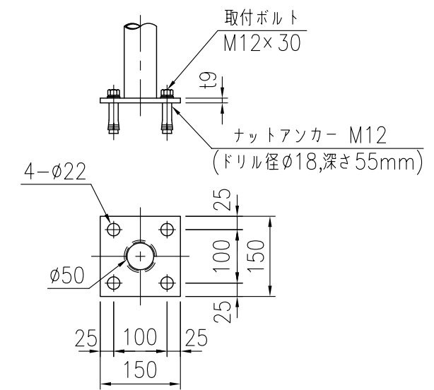
ベースプレート詳細図 (1/10)
