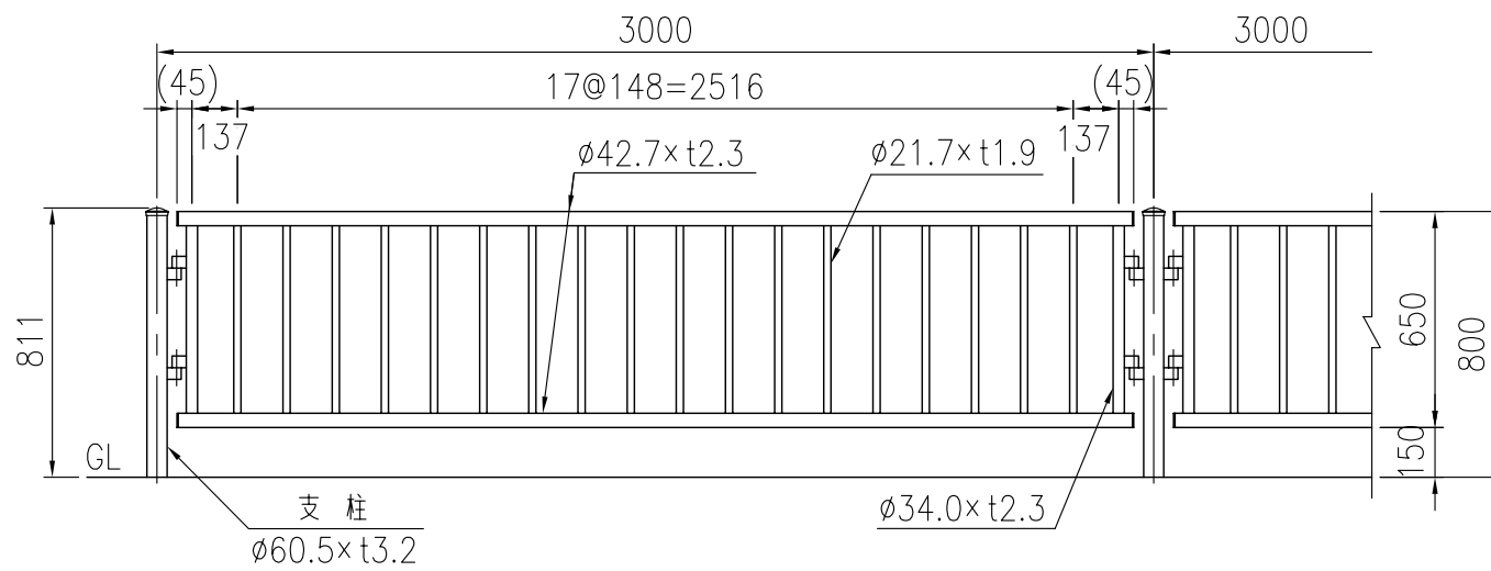
設置図 (1/25)
