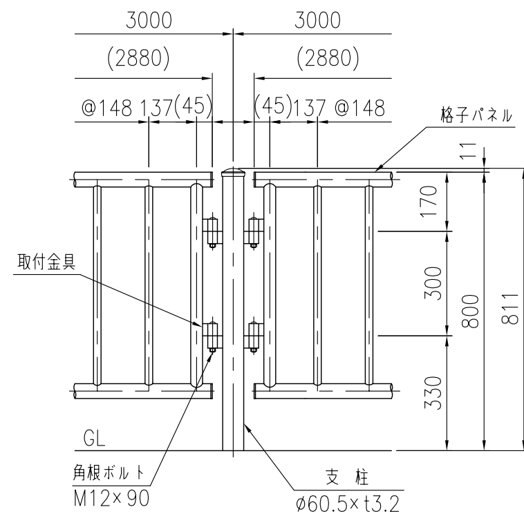
支柱図 (1/15)
