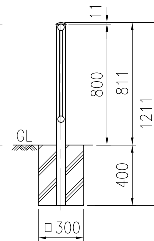
取付部詳細図 (1/4)
