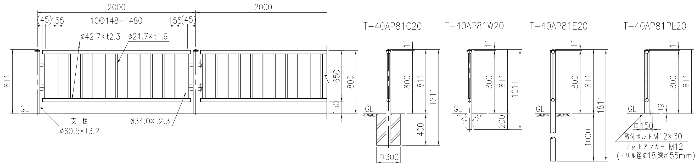
設置図 (1/25)
