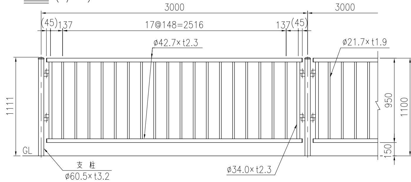
設置図 (1/25)
