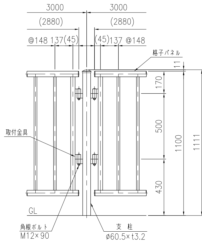
支柱図 (1/15)
