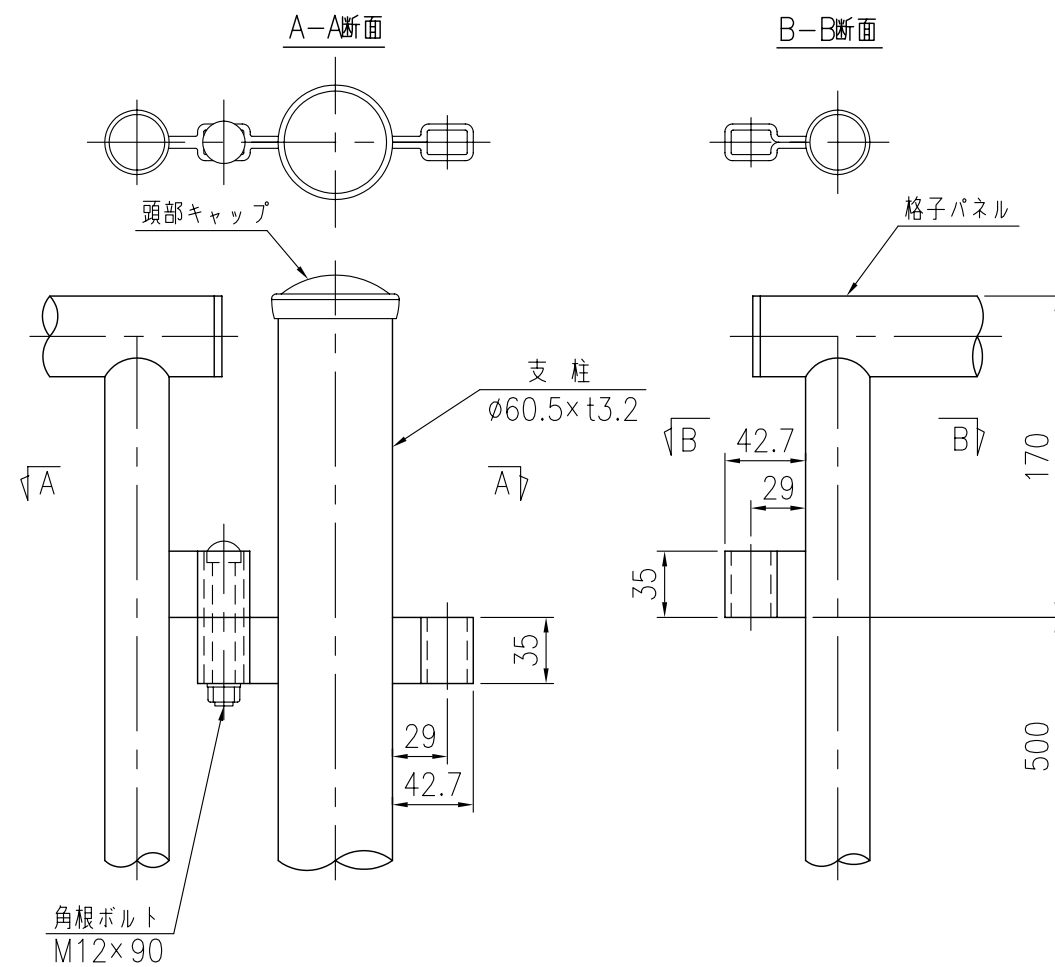
取付部詳細図 (1/4)
