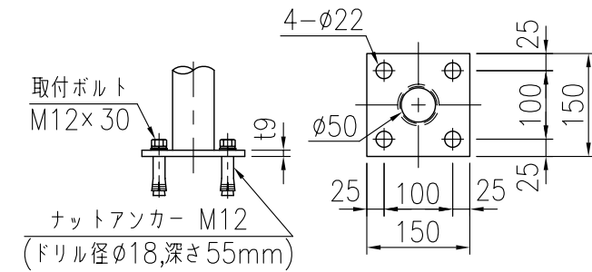
ベースプレート詳細図 (1/10)
