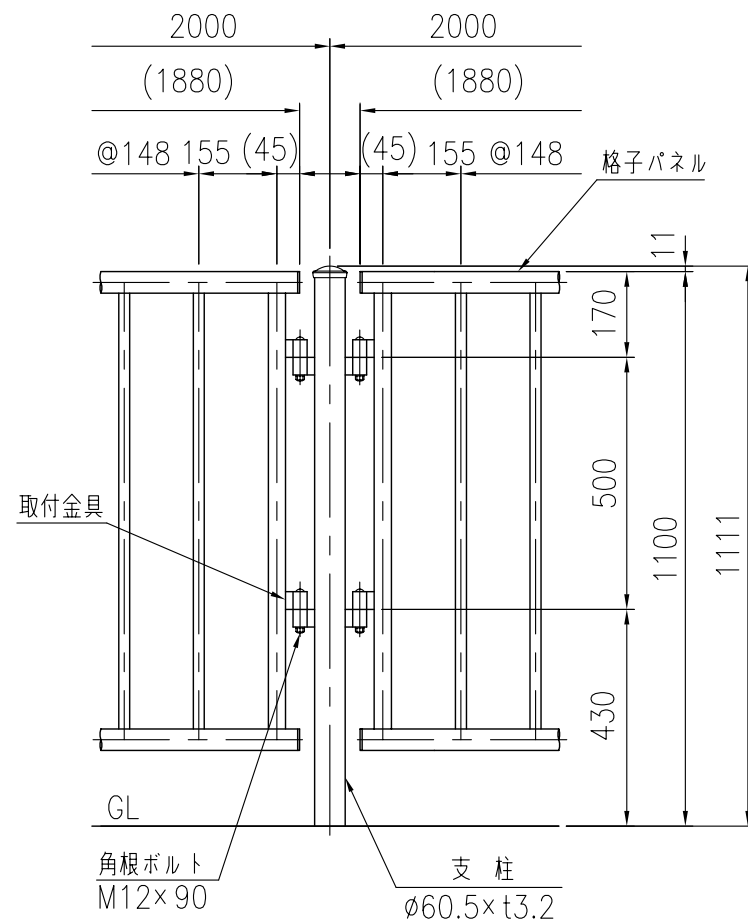
支柱図 (1/15)
