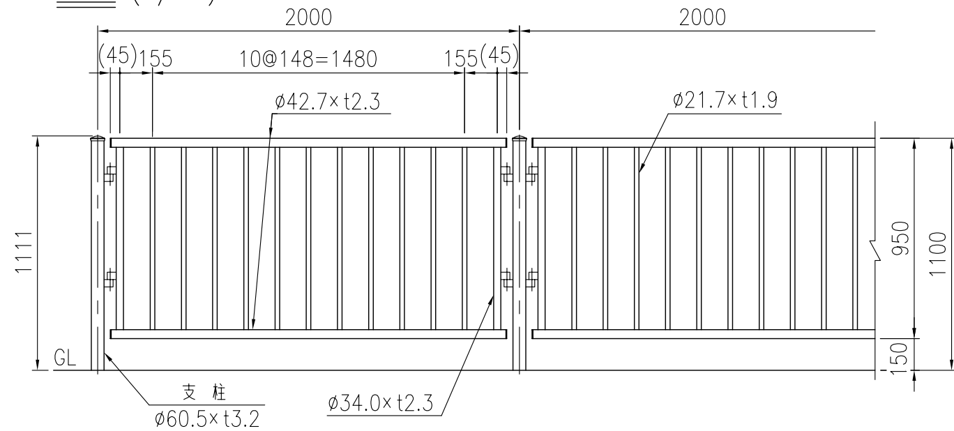
設置図 (1/25)
