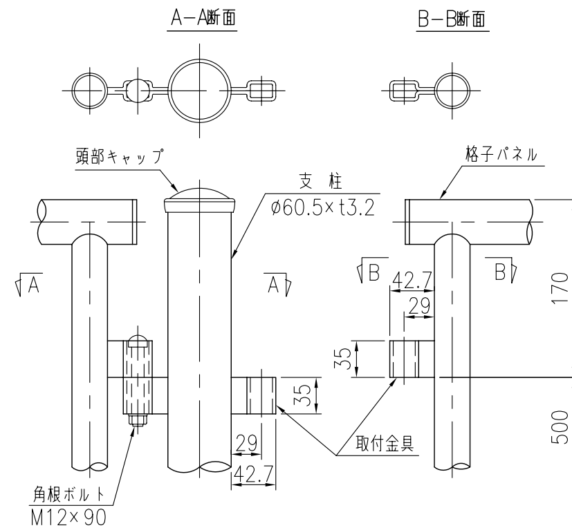
取付部詳細図 (1/5)
