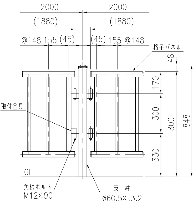
支柱図 (1/15)
