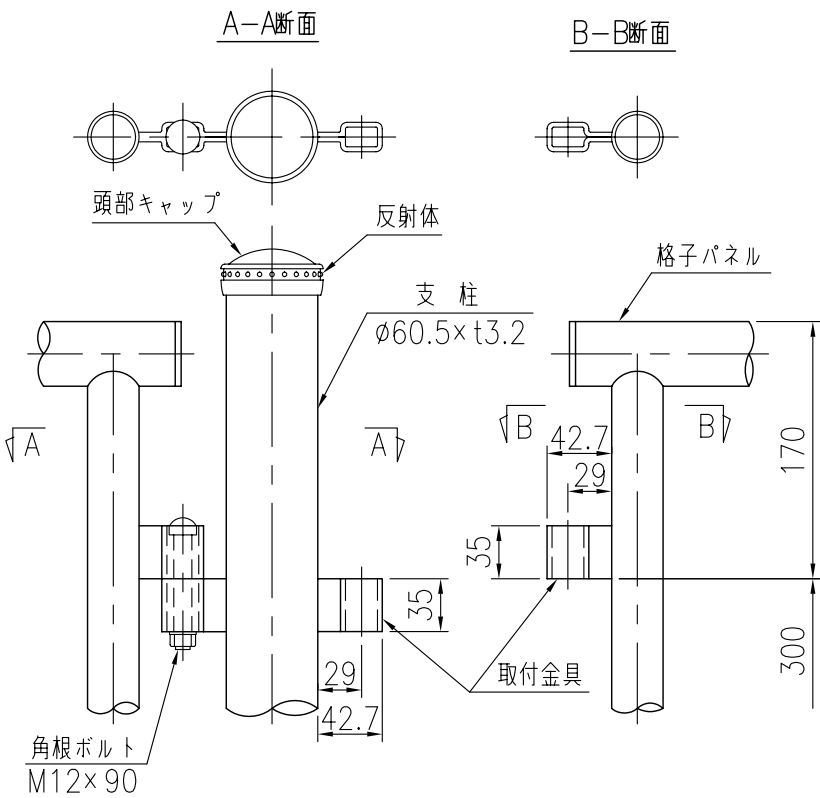
取付部詳細図 (1/4)
