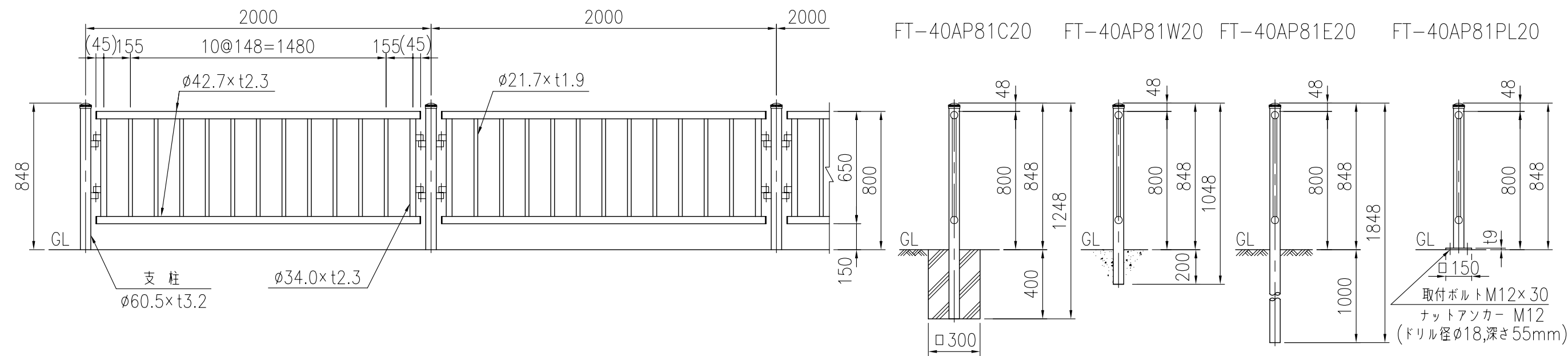
設置図 (1/25)
