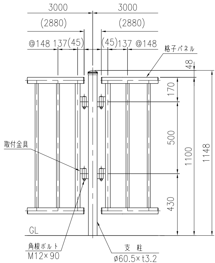
支柱図 (1/15)
