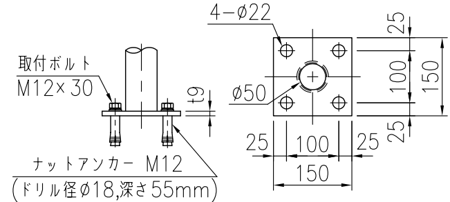
ベースプレート詳細図 (1/10)
