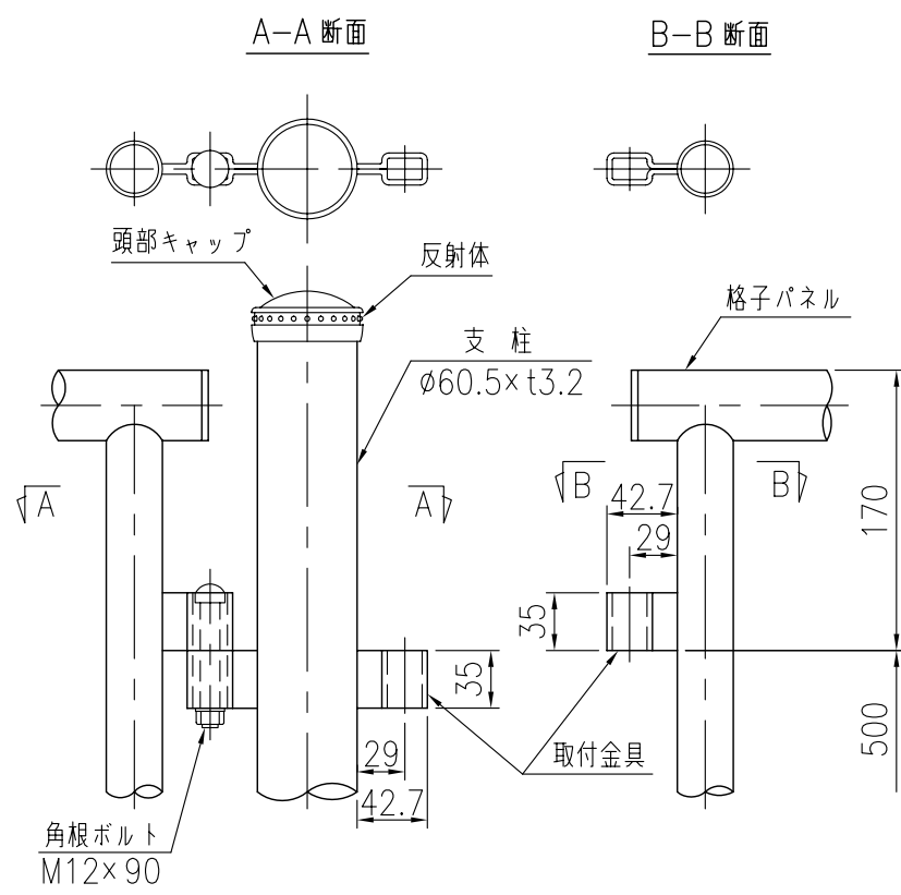
取付部詳細図 (1/4)
