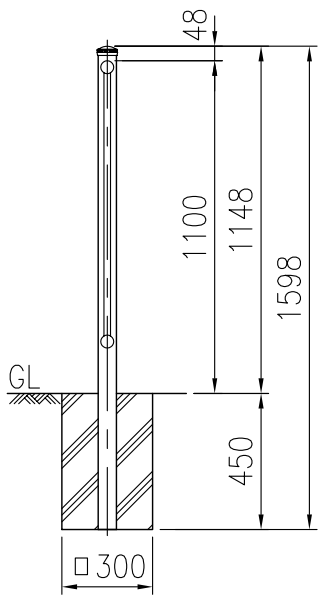
FT-40AP111C20
