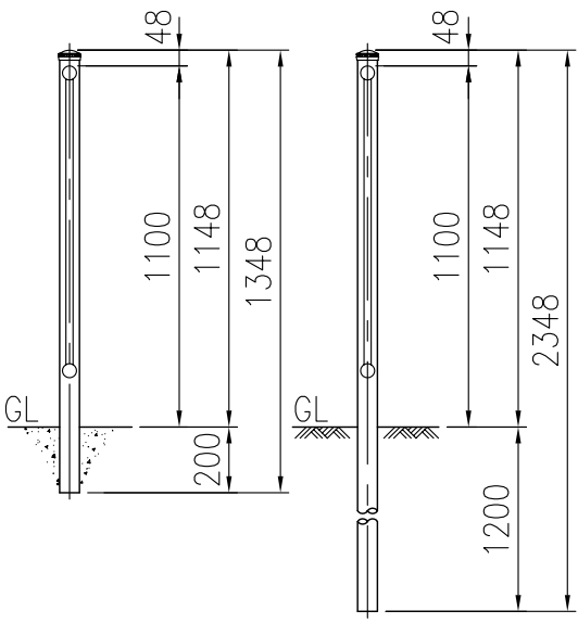
FT-40AP111E20 FT-40AP111W20
