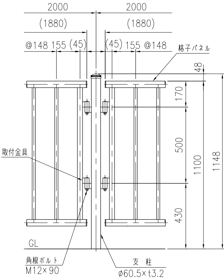
支柱図 (1/15)
