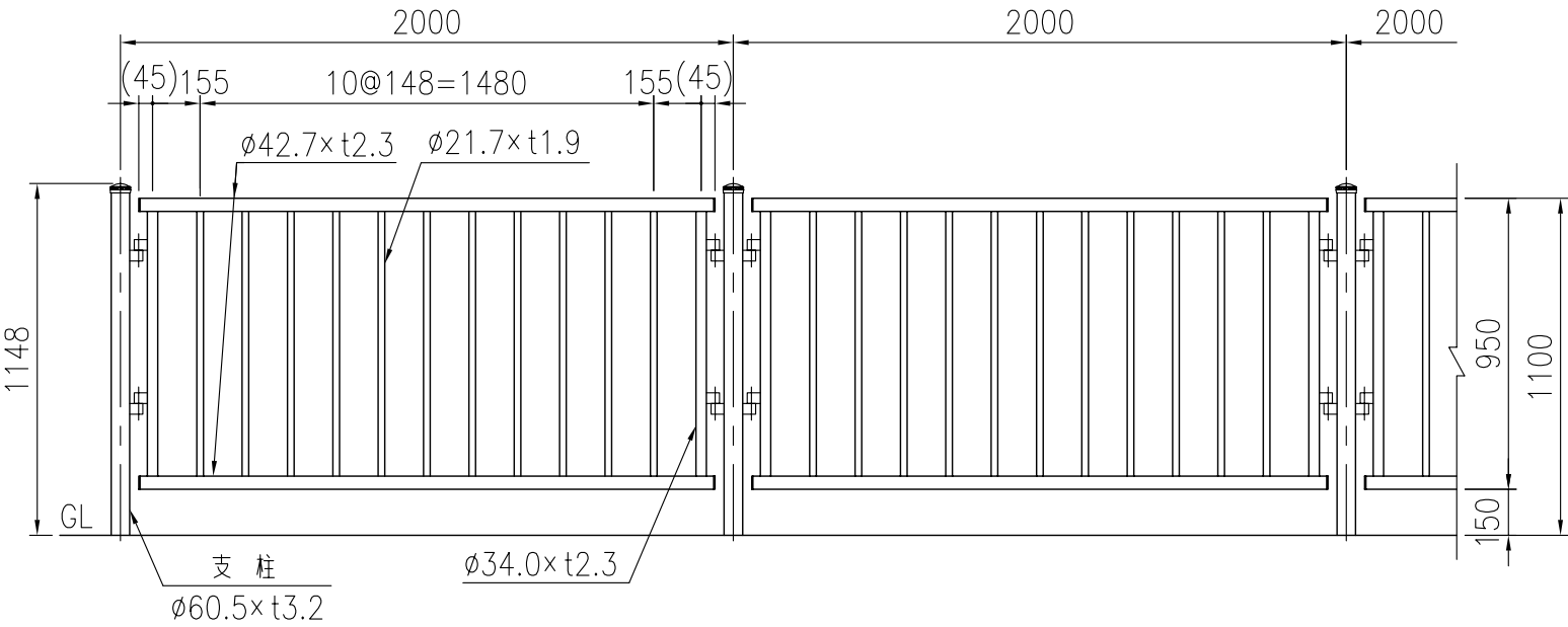
設置図 (1/25)
