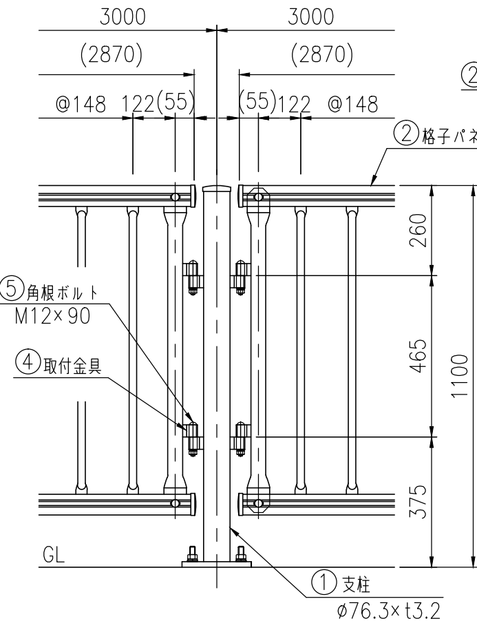
支柱図 (1/15)
