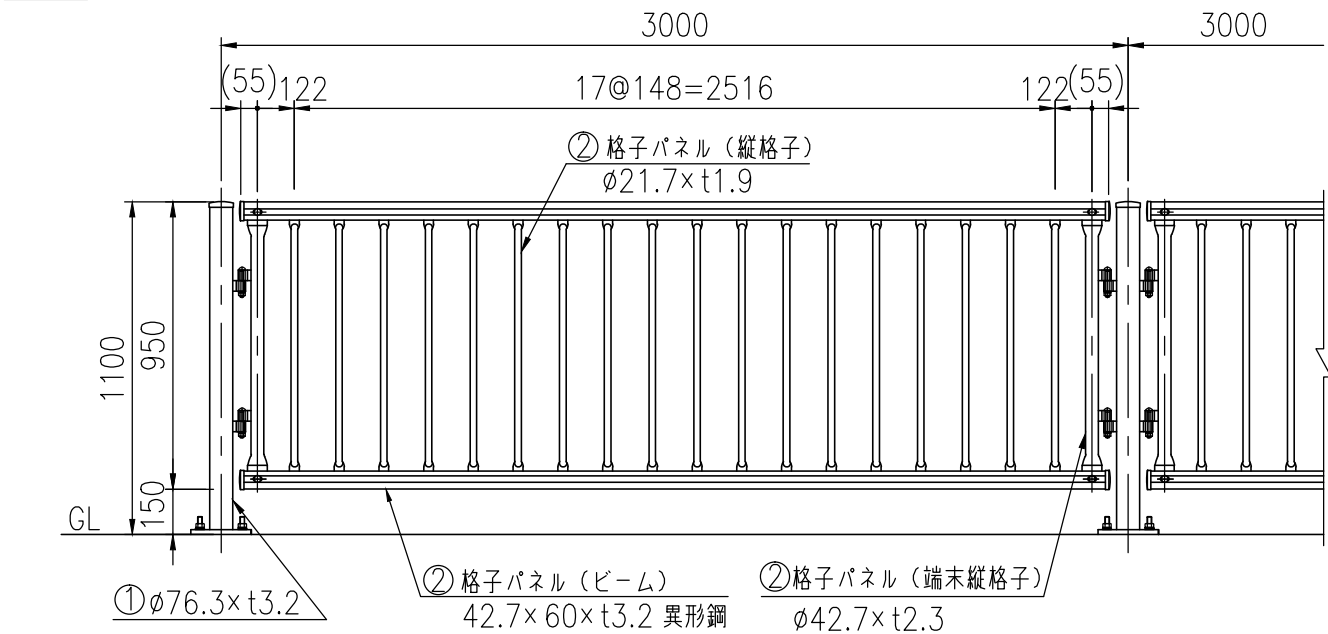
設置図 (1/25)
