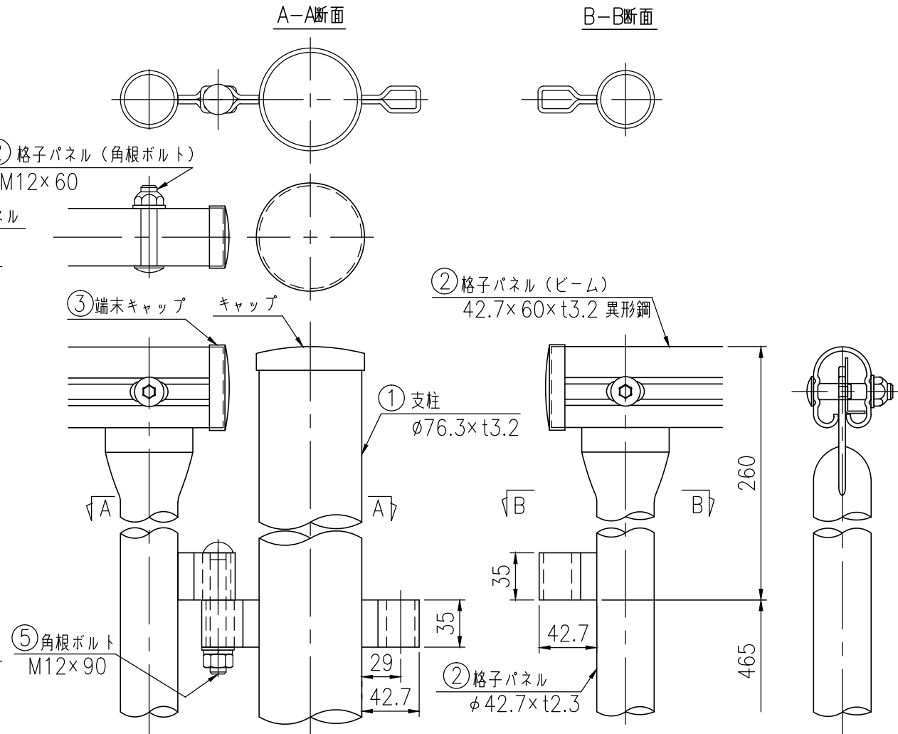
取付部詳細図 (1/4)
