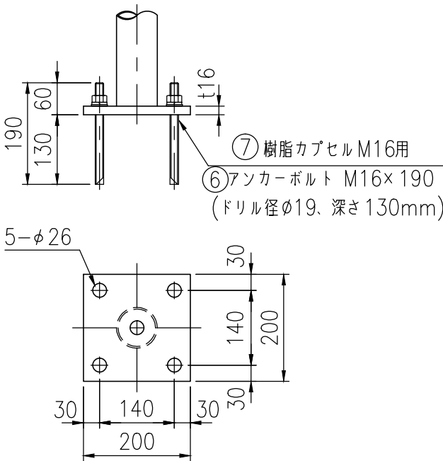
ベースプレート詳細図 (1/10)
