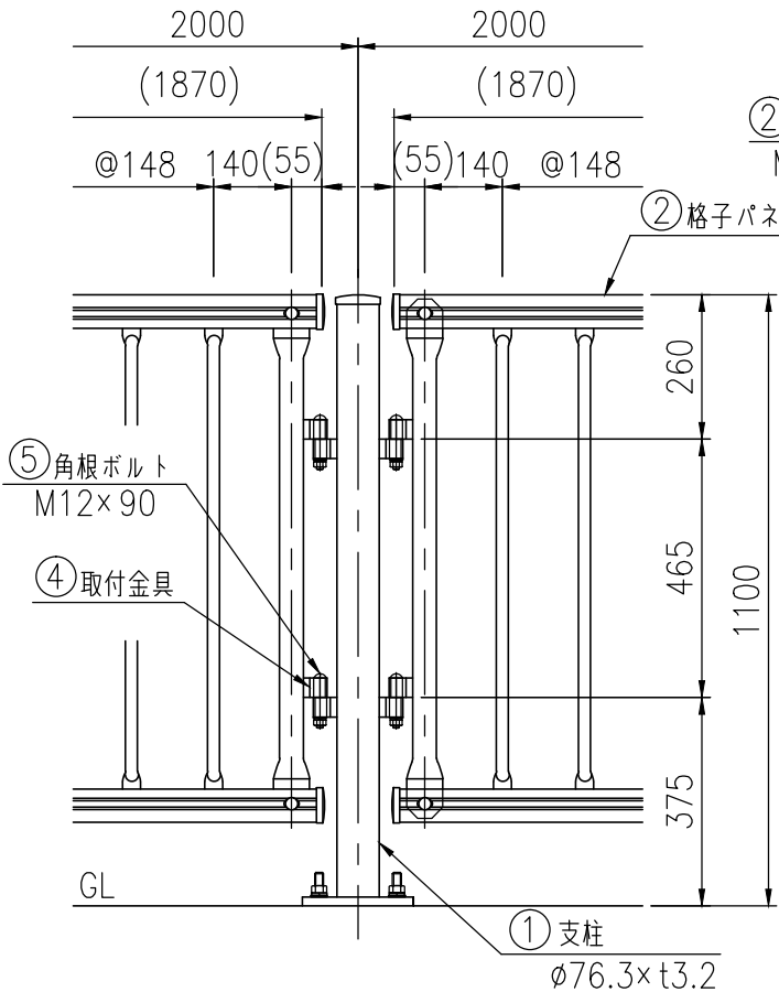
支柱図 (1/15)
