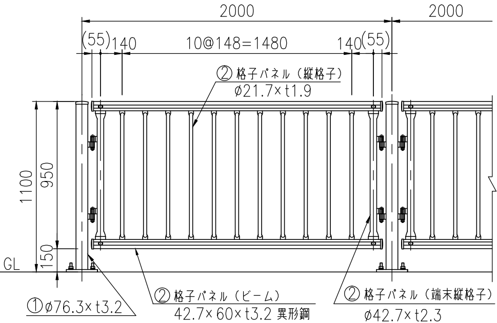
設置図 (1/25)
