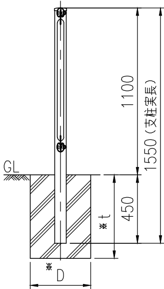
取付部詳細図 (1/4)
