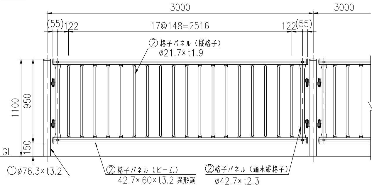
設置図 (1/25)
