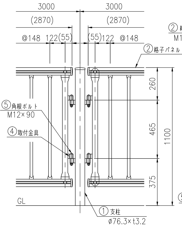
支柱図 (1/15)
