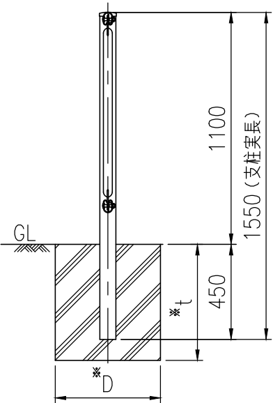
取付部詳細図 (1/4)
