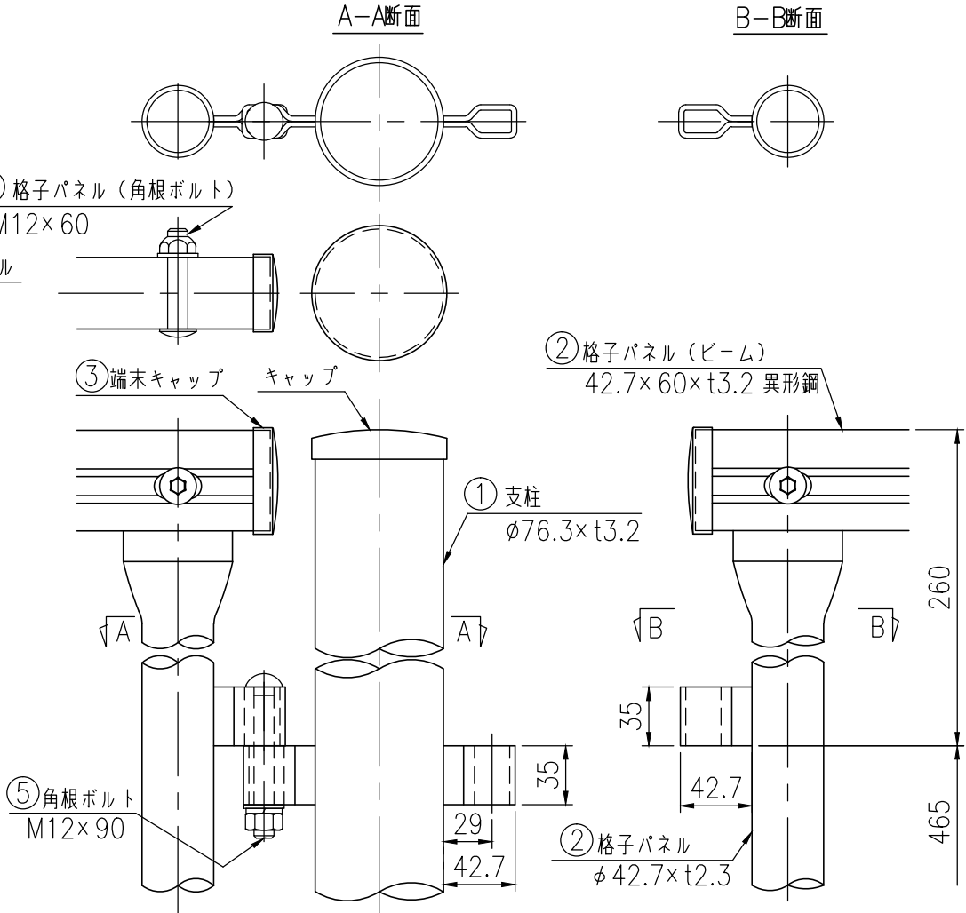
取付部詳細図 (1/4)
