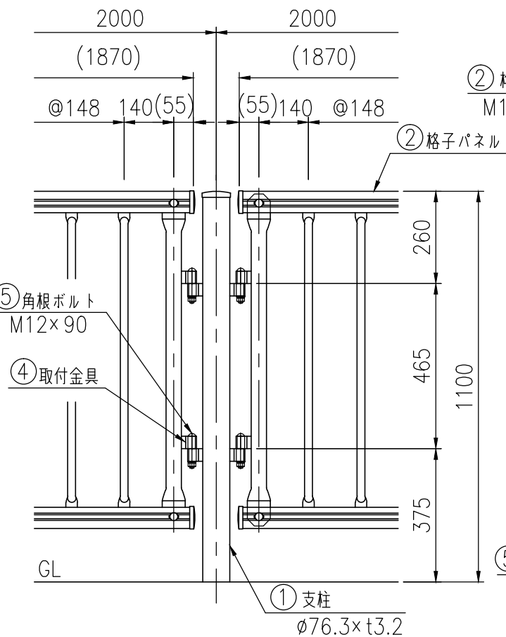
支柱図 (1/15)
