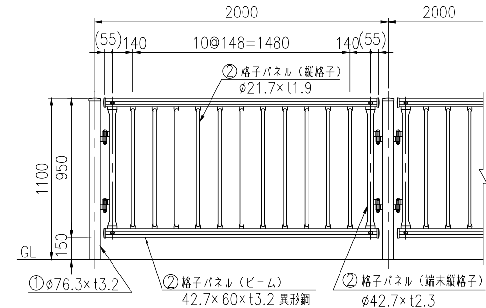
設置図 (1/25)
