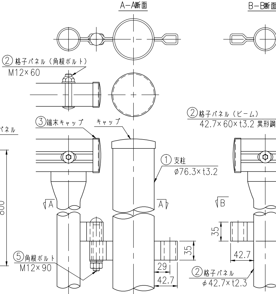
取付部詳細図 (1/4)
