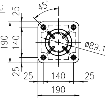
ベースプレート詳細図 (1/10)
