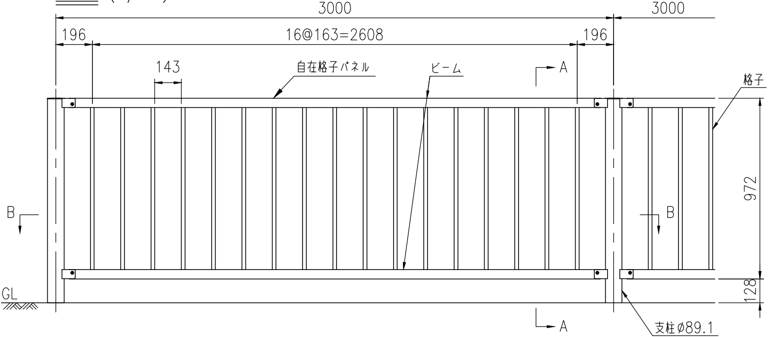
設置図 (1/20)
