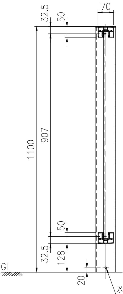
A-A断面
