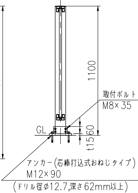
ベースプレート詳細図 (1/10)
